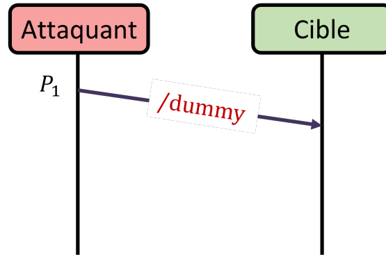
Figure 2.1: Exemple d'anomalie sémantique : une requête HTTP/2 avec une url non spécifié dans les standards qui pourrait être le résultat d'une attaque de fuzzing.
