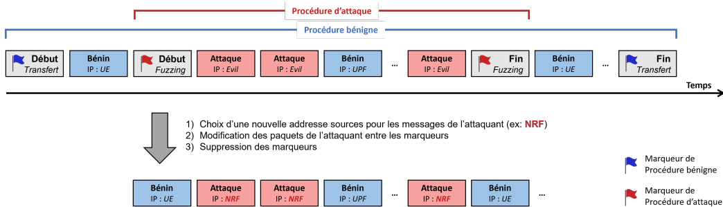
Figure 5.2: Processus de labellisation préservant les contextes temporels et topologiques grâce à l'utilisation de marqueurs.
