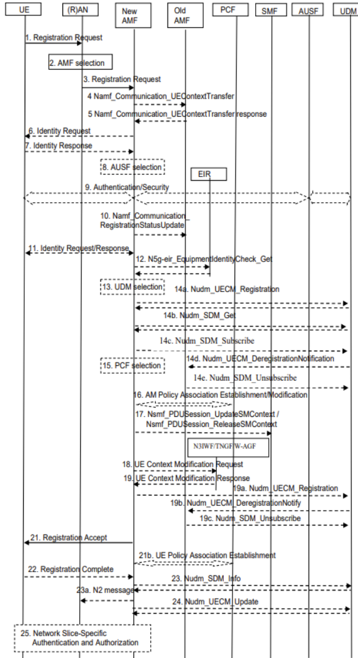
Figure 5.1: Procédure générale d'enregistrement tel que proposé dans la TS 23.502 de 3GPP[?].
