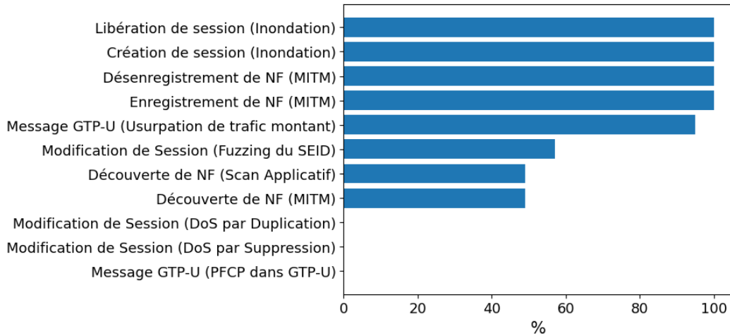
Figure 5.3: Proportion de messages bénins sémantiquement identiques à des messages d'attaque de même nature.
