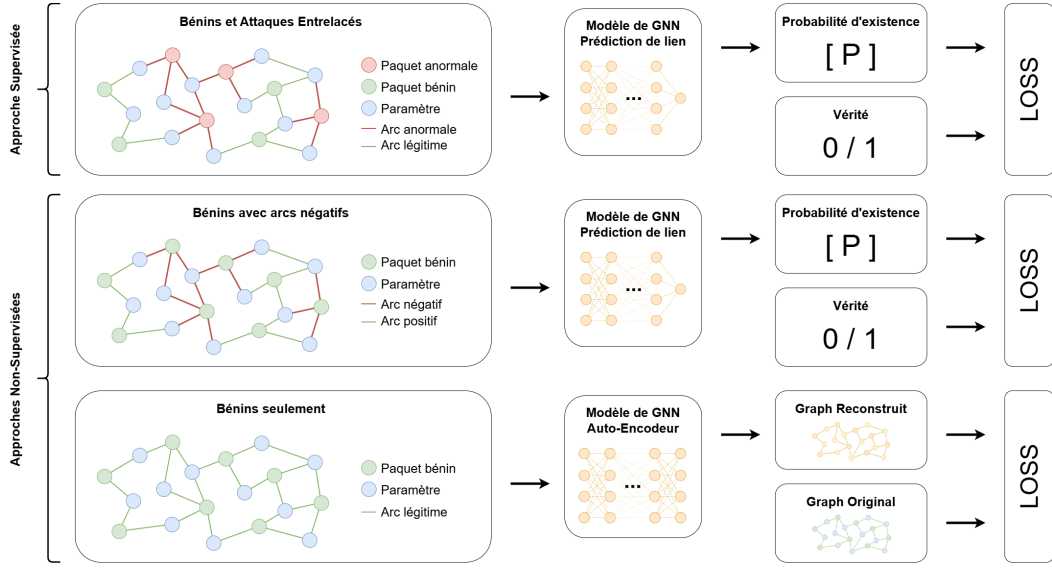
Figure 5.6: Comparaison des différentes approches d'apprentissage : (a) approche supervisée avec des données annotées, (b) approche non supervisée basée sur la prédiction de liens, et (c) approche non supervisée basée sur un autoencodeur.
