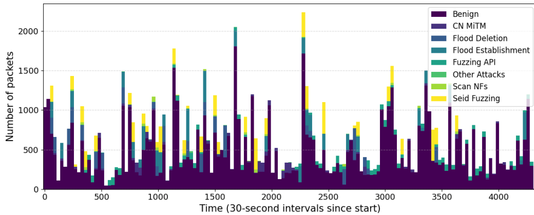
Figure 5.4: Distribution des messages issues de procédures d'attaques et bénignes en fonction du temps.
