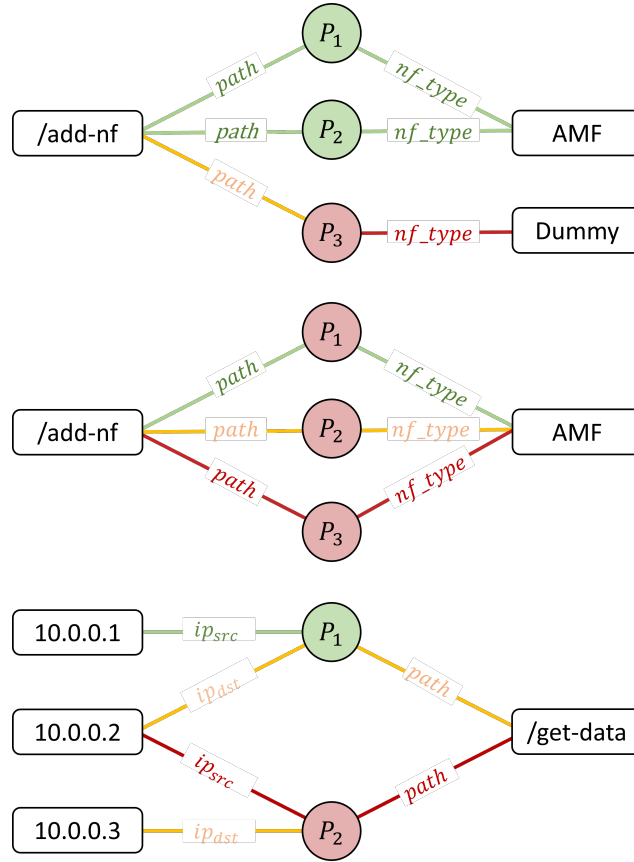
Figure 5.7: Représentation des coefficients d'anomalies pour les dimensions (a) sémantique, (b) séquentielle, et (c) topologique. Les noeuds rouges représentent des paquets d'attaque tandis que les verts représentent des paquets bénins.
