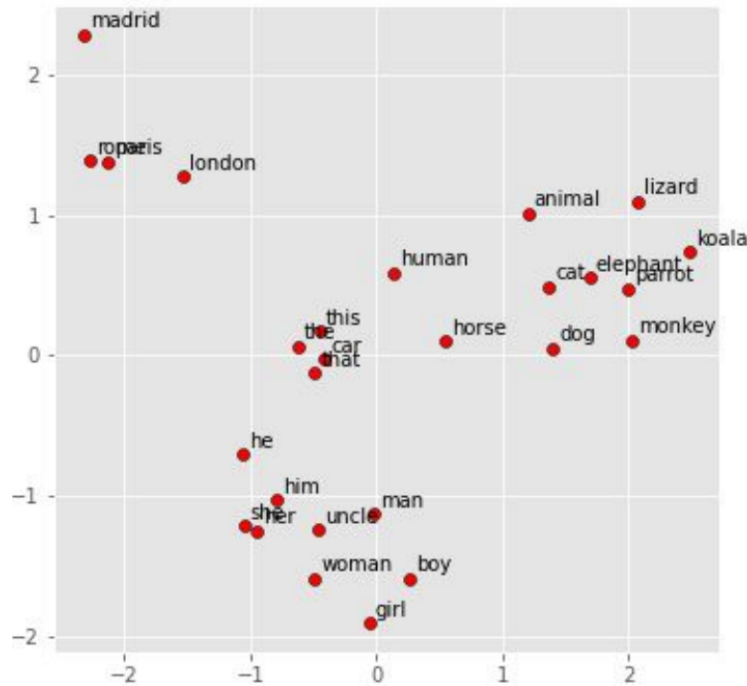
Figure 3.13: Projection en deux dimensions d'un espace latent représentant un vocabulaire anglais, obtenue par analyse en composantes principales (PCA).
