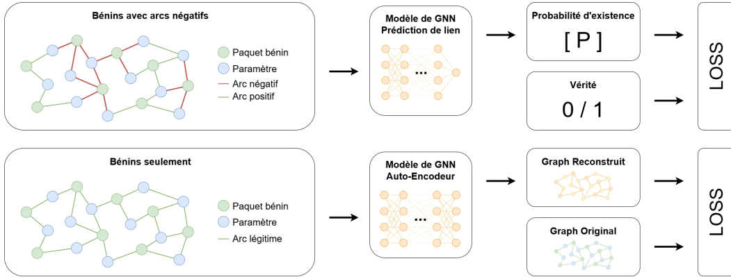
Figure 1.7: Représentation du processus d'apprentissage non supervisé. La première ligne correspond à une tâche de prédiction de lien avec des arcs négatifs artificiels, tandis que la seconde ligne correspond à une tâche de reconstruction.
