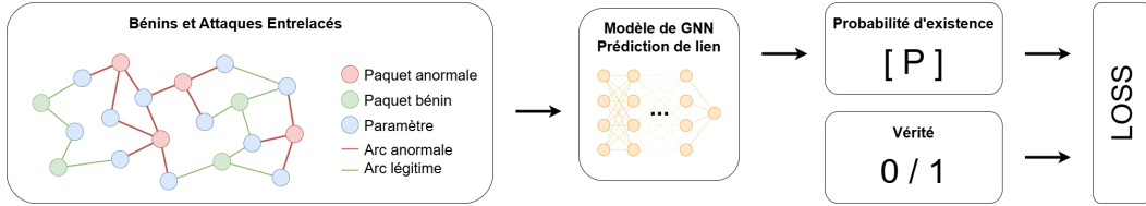
Figure 1.6: Représentation du processus d'apprentissage supervisé.
