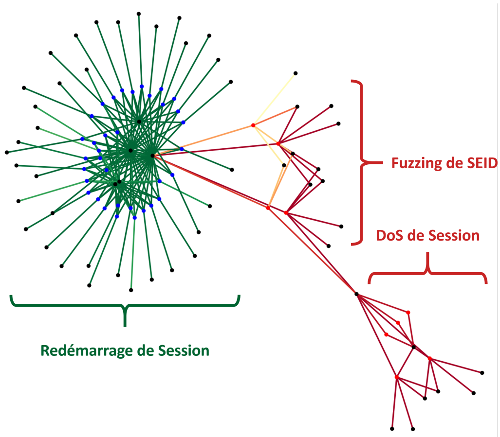
Figure 1.9: Représentation de la prédiction d'anomalie sur un graph représentant un ensemble de paquets observés. Les arcs rouges signalent des anomalies très probables tandis que les arcs verts signalent une faible probabilité d'anomalie. Les paquets bénins sont représentés comme des nœuds de couleur bleu et les paquets d'attaques comme des nœuds de couleur rouge.
