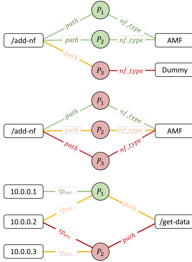
Figure 1.8: Représentation des coefficients d'anomalies pour les dimensions (a) sémantique, (b) séquentielle, et (c) topologique. Les nœuds rouges représentent des paquets d'attaque tandis que les verts représentent des paquets bénins.
