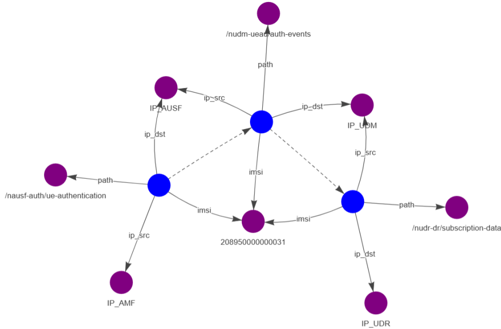
Figure 3.11: Représentation sous forme de graphe d'une procédure composée de trois paquets. Les arcs orientés en pointillés représentent un nouveau type de liaison entre nœuds central permettant de représenter l'ordre temporel des échanges.
