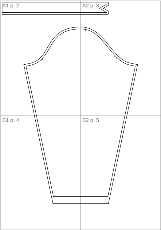
Manche + Bande d'encolure
