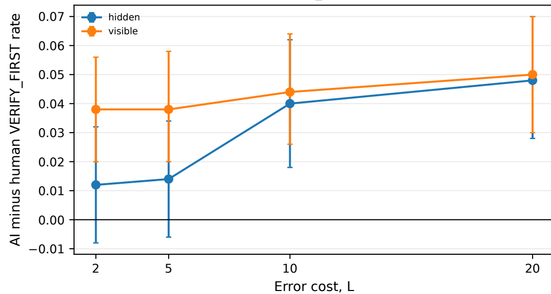
openai_gpt56_sol
