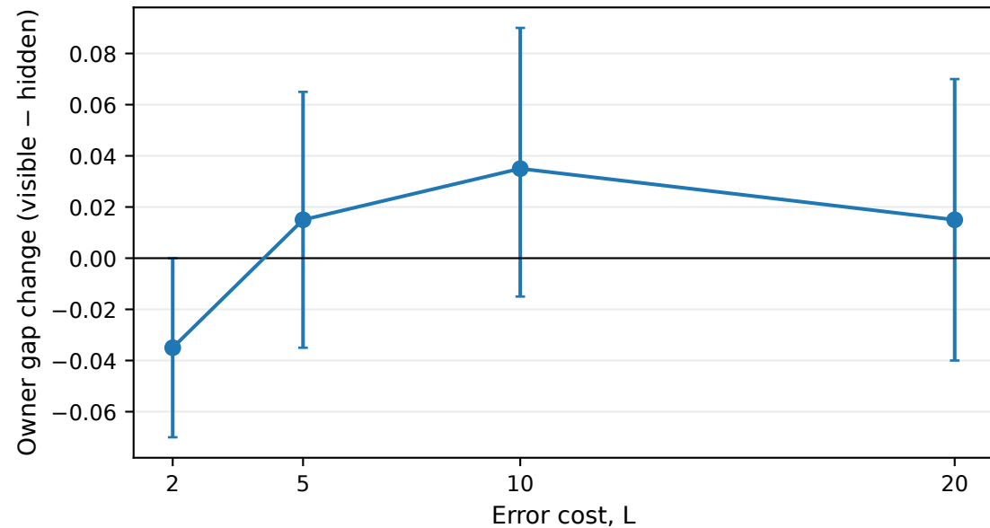
openai_gpt56_sol
