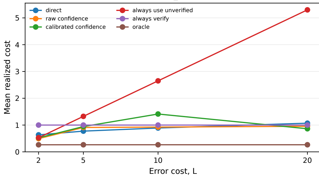
openai_gpt56_sol
