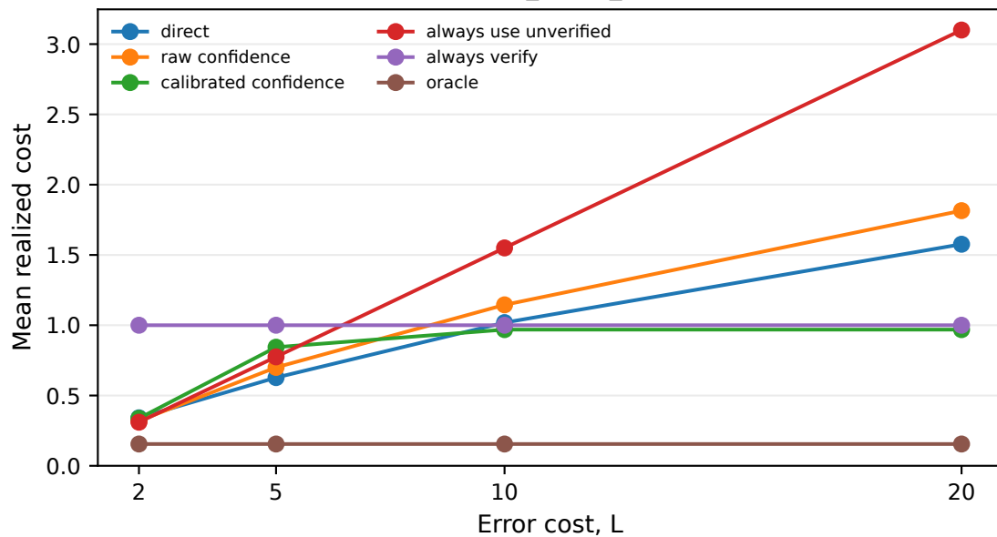
openai_gpt56_sol
