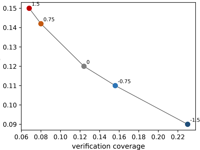
GPT MMLU-Pro
