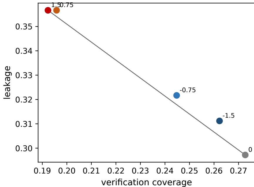
GPT LiveCodeBench
