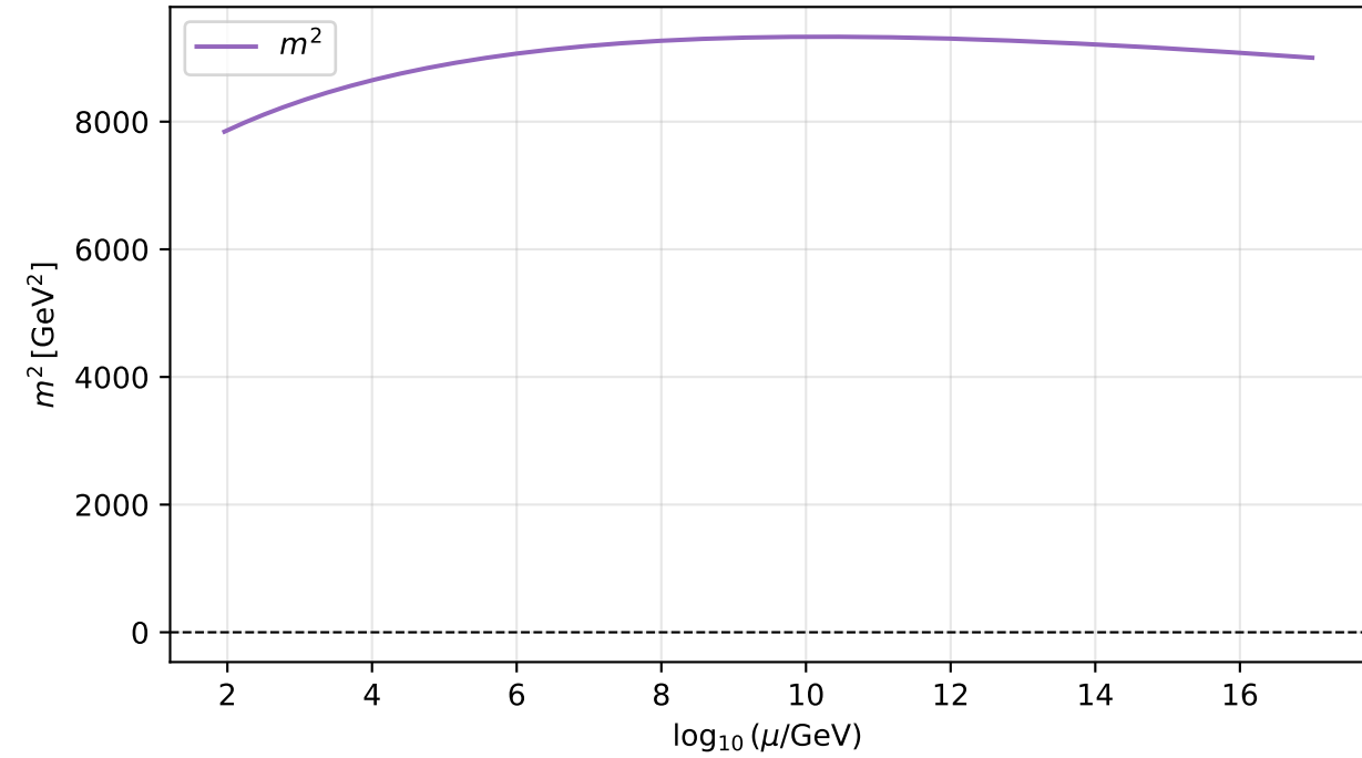
Higgs mass parameter
