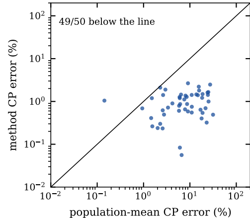
Levenberg-Marquardt
