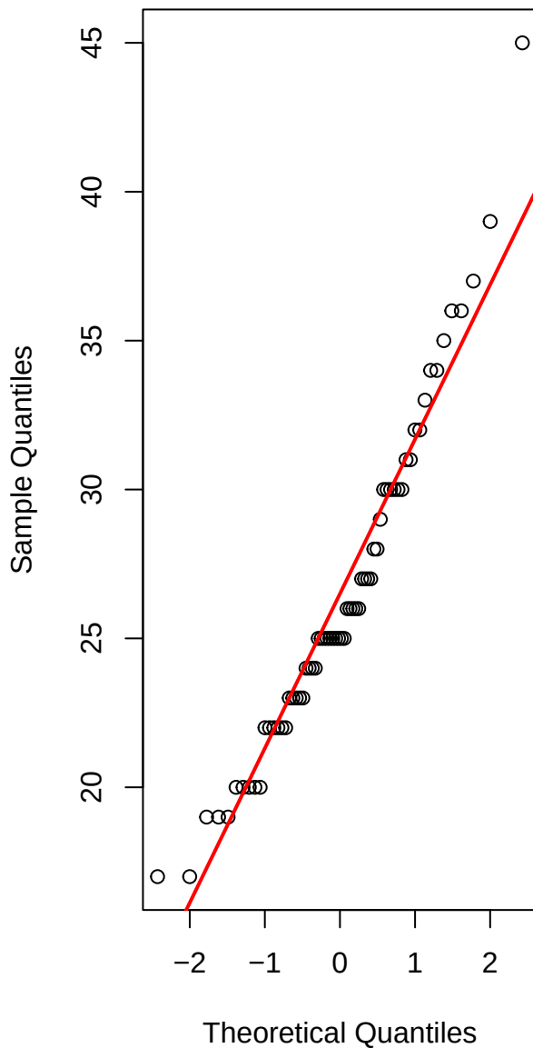
Q-Q plot du BMI
