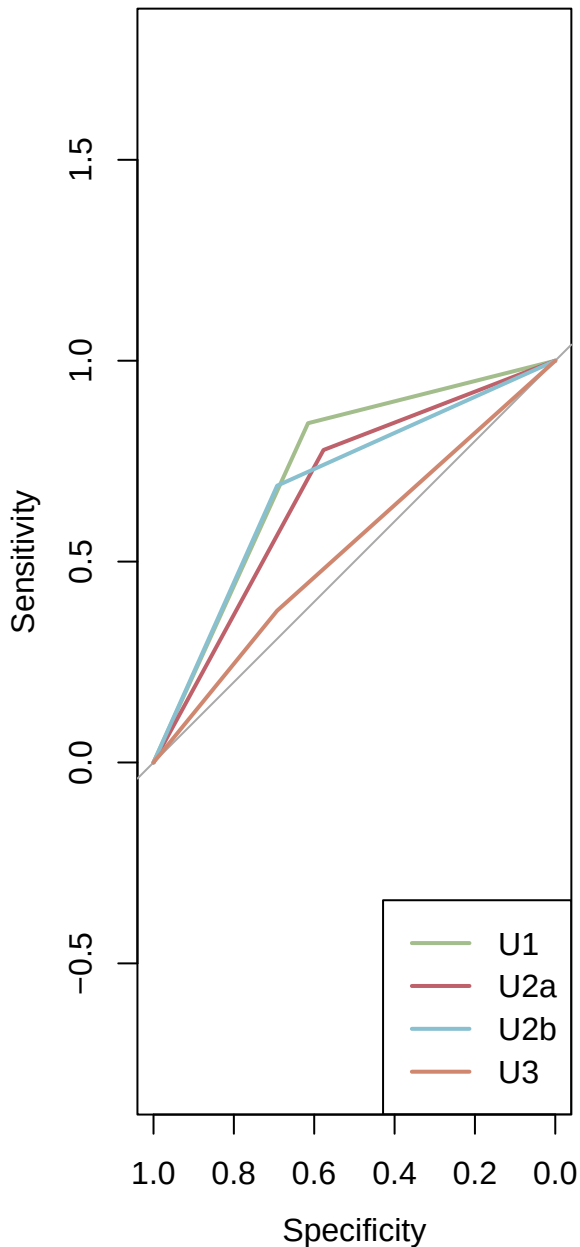
Courbes ROC comparées
