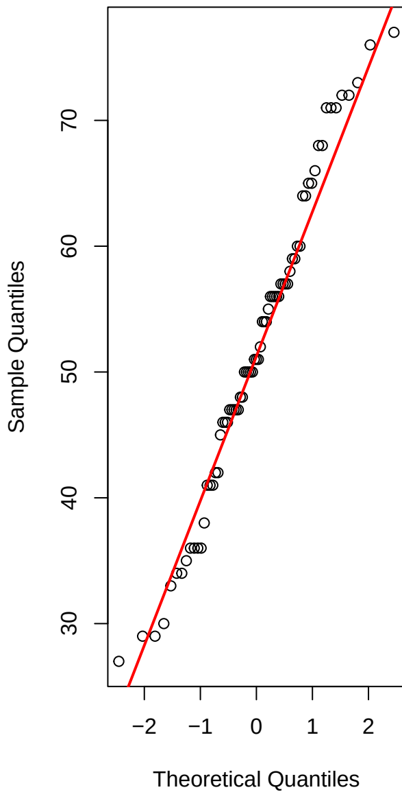
Q-Q plot de l'âge
