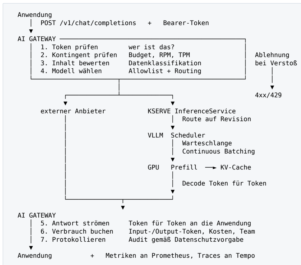
Der Weg einer Anfrage, mit den Entscheidungen an jeder Station
