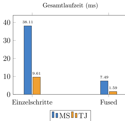
Abbildung 12: Fused Pipeline vs. Summe der isolierten Einzelschritte für MS- und TJ-Messungen.
