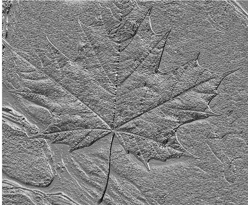
Abbildung 7: Ausschnitt des Sobel-Outputs der Gradientenrichtungen, die von Radians auf den Wertebereich 0-255 übertragen wurden.
