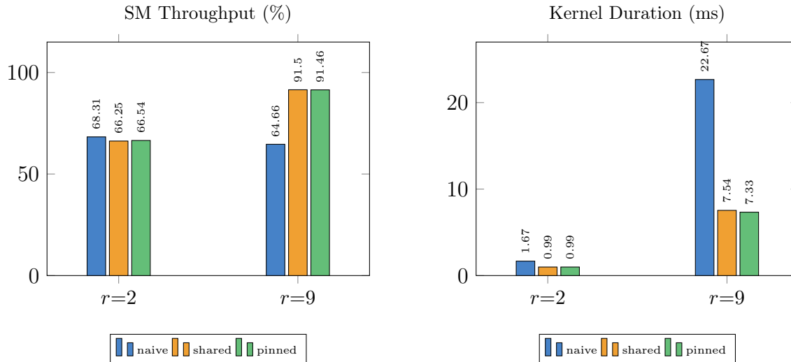
Abbildung 4: NCU-Profilung, Vergleich naive/shared/pinned bei r=2 und r=9 (200 Runs Avg).
