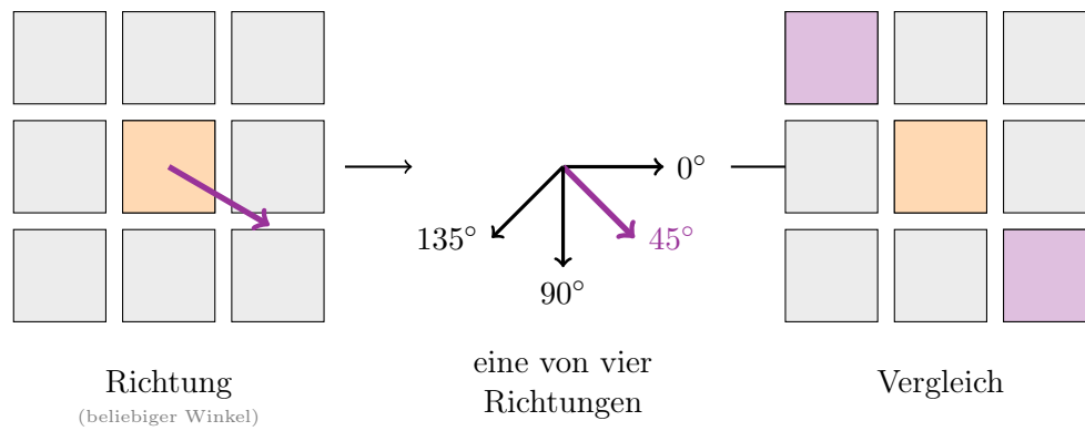
Abbildung 5: Non-Maximum Suppression: Die Gradientenrichtung wird auf eine von vier Achsen quantisiert ( 0^\circ , 45^\circ , 90^\circ , 135^\circ ). Anschließend wird der Pixel mit den beiden farbig markierten Nachbarn entlang der gewählten Achse verglichen.
