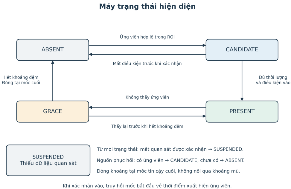
Hình 9 Luồng cài đặt máy trạng thái hiện diện
