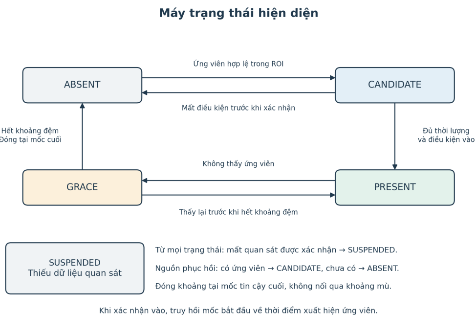
Hình 3 Máy trạng thái hiện diện đề xuất
