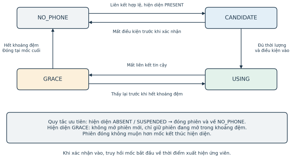
Hình 4 Máy trạng thái sử dụng điện thoại đề xuất
