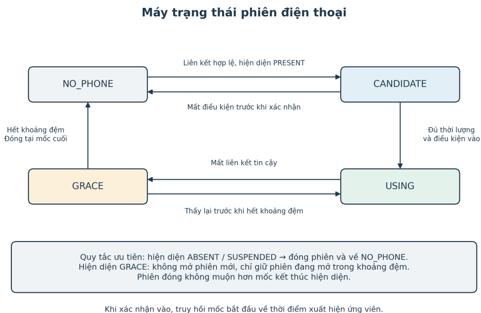
Hình 10 Luồng cài đặt máy trạng thái sử dụng điện thoại
