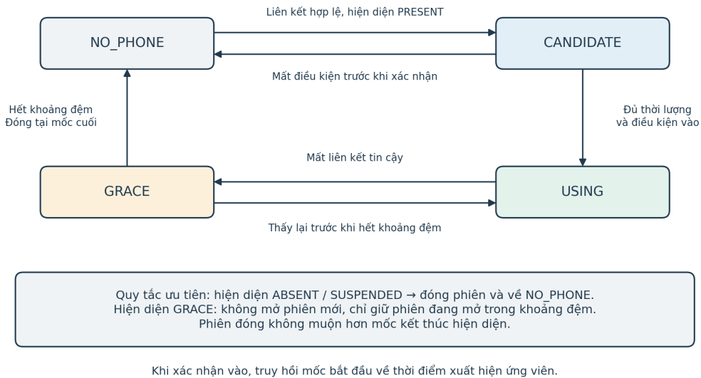
Hình 8 Máy trạng thái theo dõi phiên sử dụng điện thoại
