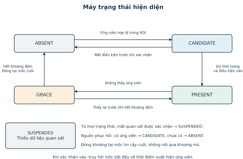
Hình 7 Máy trạng thái hiện diện ở cấp nhân viên
