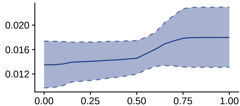
2y YLD
