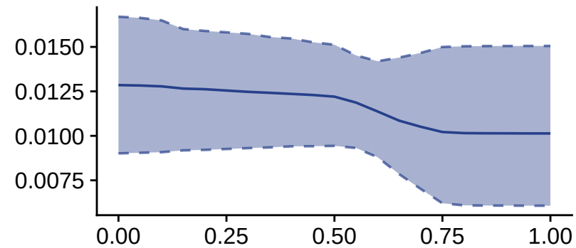
6y YLD
