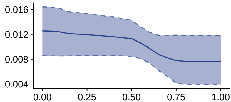
8y YLD
