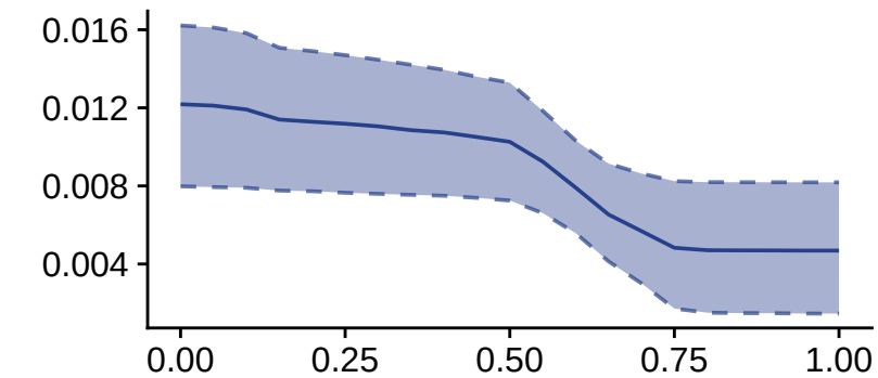
12y YLD
