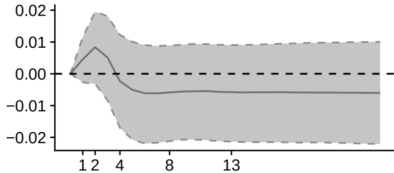
2y YLD
