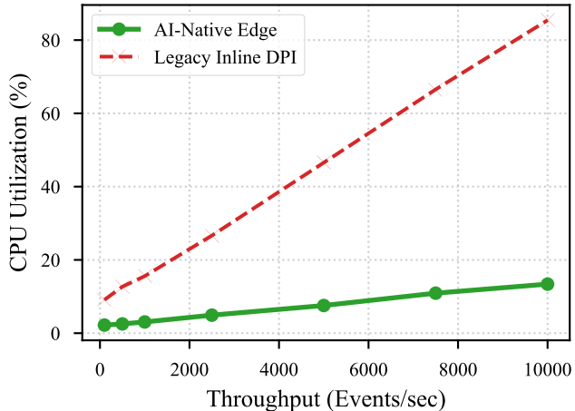
Edge CPU Overhead
