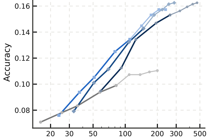
AMC23
