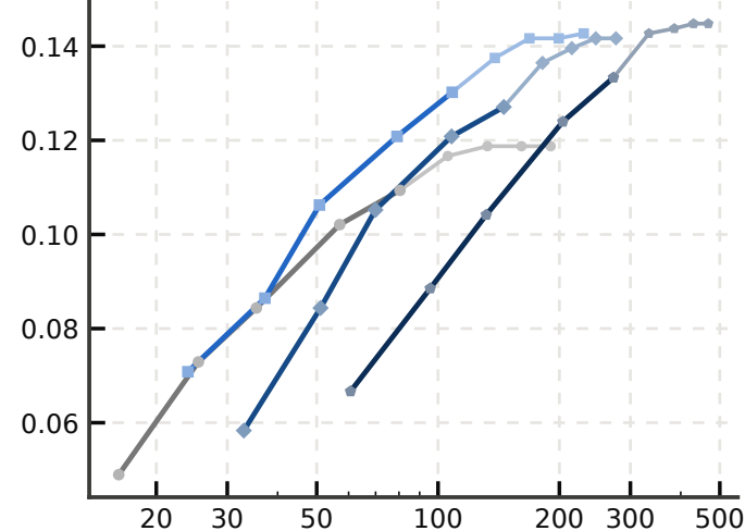
OlympiadBench
