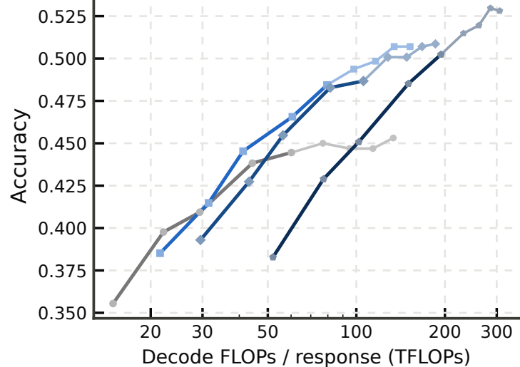
AMC23
