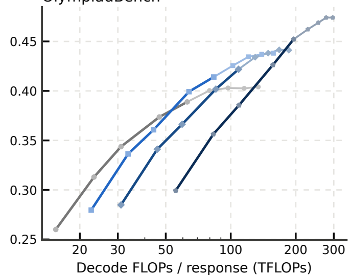
OlympiadBench
