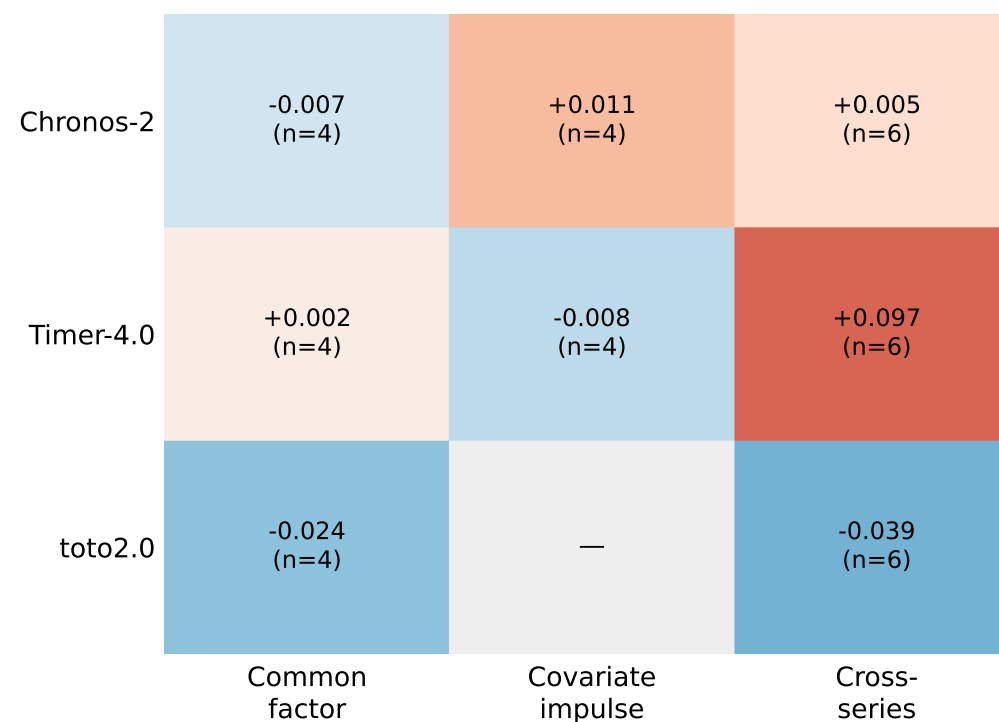
FEV-Mini20
