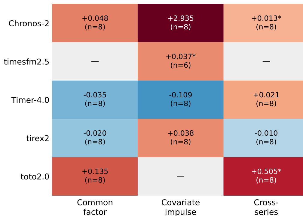
FEV-Mini20
