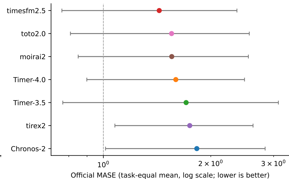
FEV-Mini20
