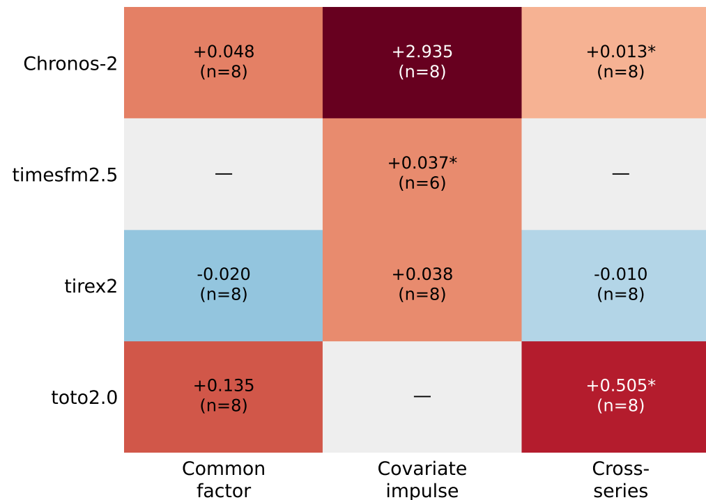
FEV-Mini20
