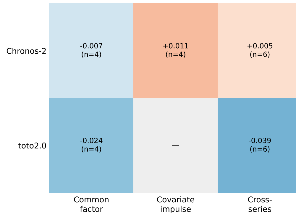
FEV-Mini20
