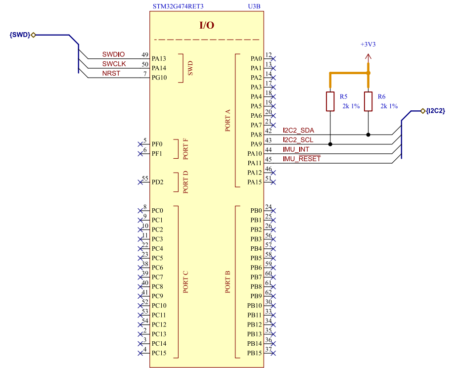
MCU GPIOs
