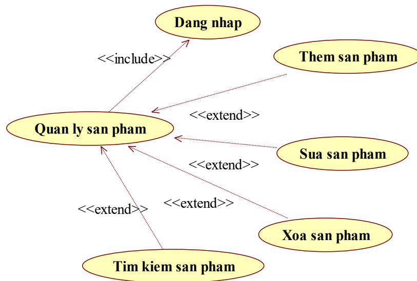
Hình 3.2.Sơ đồ phân rã chức năng quản lý sản phẩm
