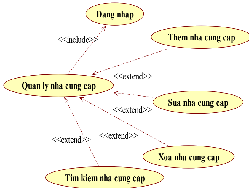
Hình 3.4. Sơ đồ phân rã chức năng quản lý nhà cung cấp
