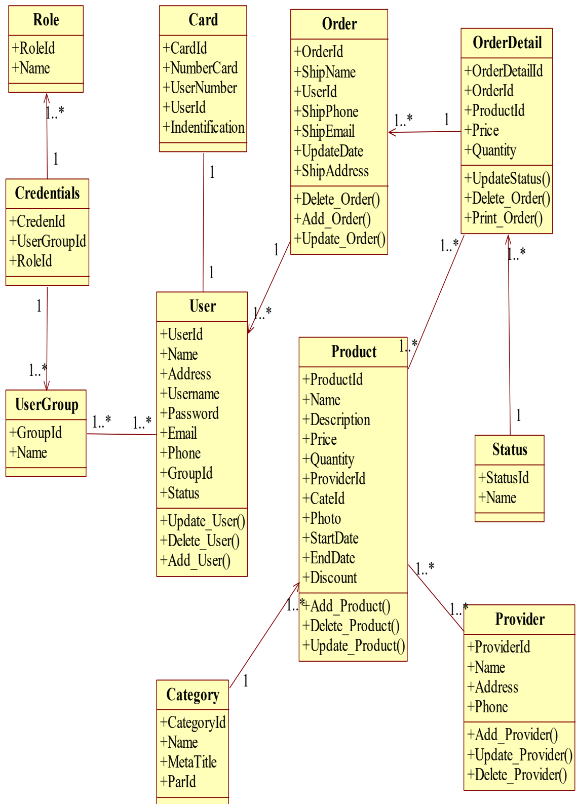
Hình 3.11. Biểu đồ lớp chi tiết hệ thống
