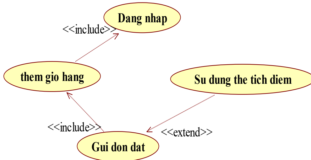
Hình 3.9. Sơ đồ phân rã chức năng gửi đơn đặt
