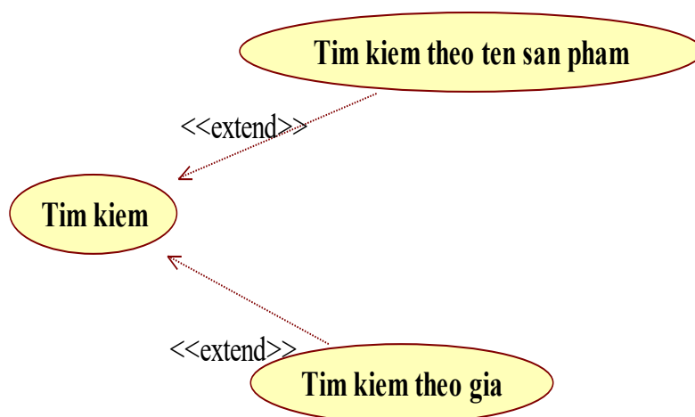
Hình 3.5. Sơ đồ phân rã chức năng tìm kiếm
