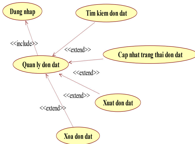
Hình 3.8. Sơ đồ phân rã chức năng quản lý đơn đặt
