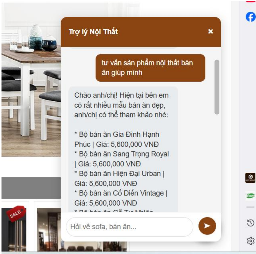
Hình 4.34. Giao diện Chatbox AI tư vấn sản phẩm
