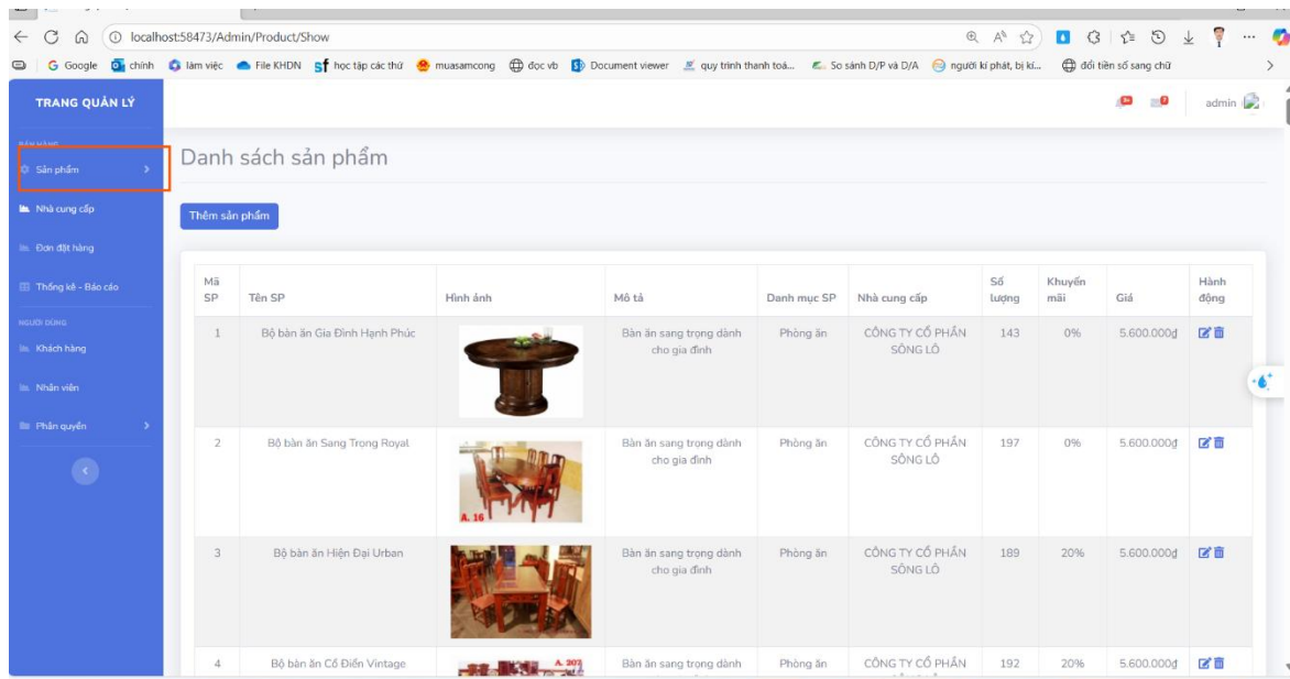
Hình 4.23. Giao diện Quản lý danh sách sản phẩm
