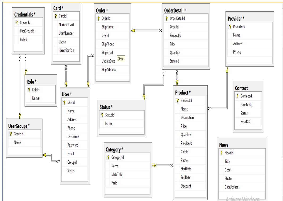
Hình 3.12. Sơ đồ ERD tổng quan hệ thống
