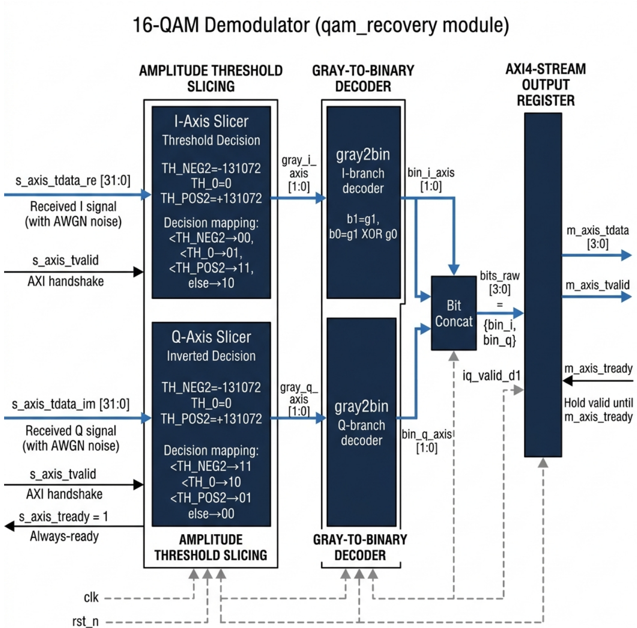
Hình 3.2: Sơ đồ khối kiến trúc RTL bộ giải điều chế 16-QAM (qam_recovery)
