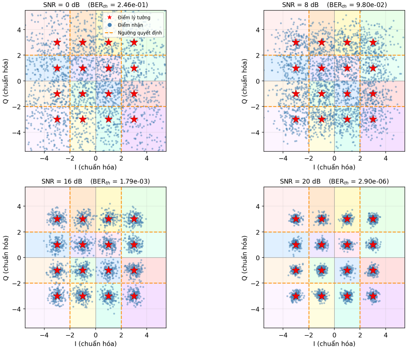
Hình 4.2: Giản đồ chòm sao 16-QAM cải tiến: nền Voronoi 16 vùng quyết định màu nhạt, điểm nhận (xanh), tâm lý tưởng (★ đỏ), ngưỡng quyết định (cam đứt nét) và BER lý thuyết BER_{th} ghi trên mỗi ô.
