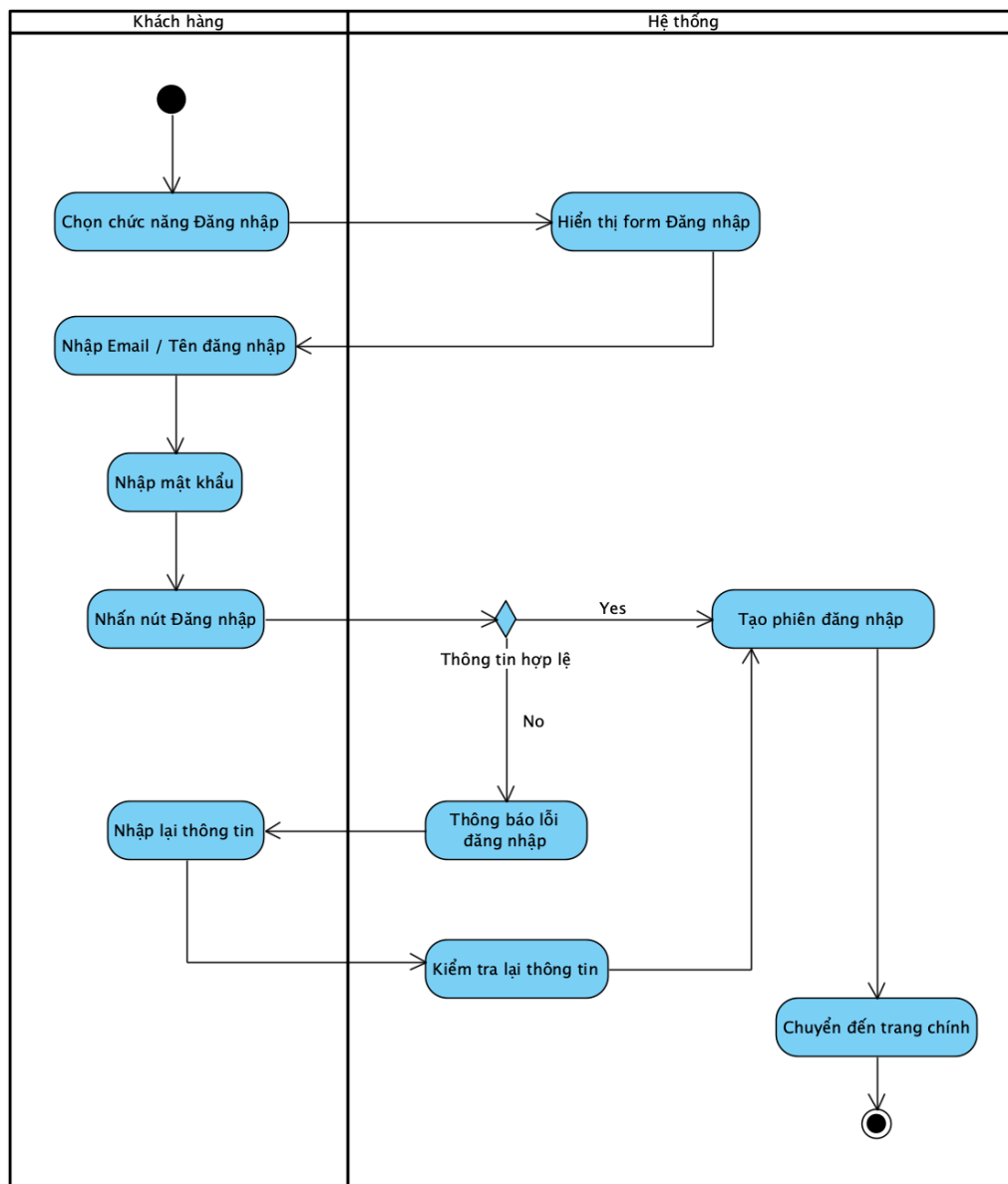
Hình 2.9: Biểu đồ hoạt động Đăng nhập tài khoản
