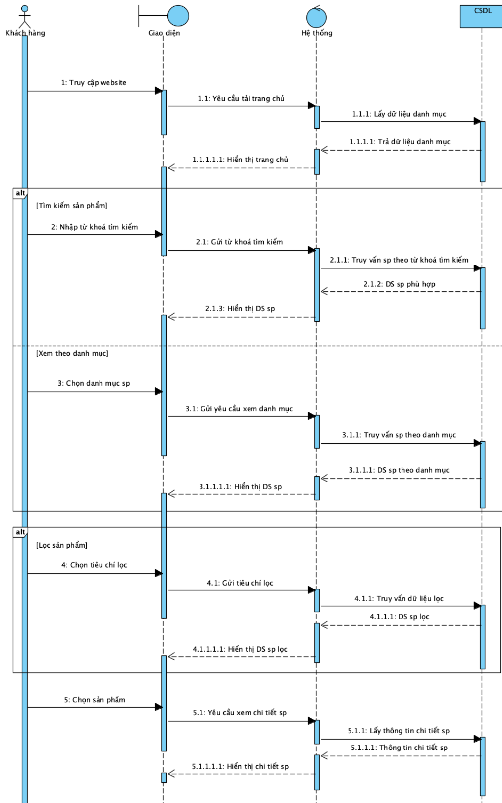
Hình 2.14: Biểu đồ tuần tự Tìm kiếm/ Xem danh sách sản phẩm
