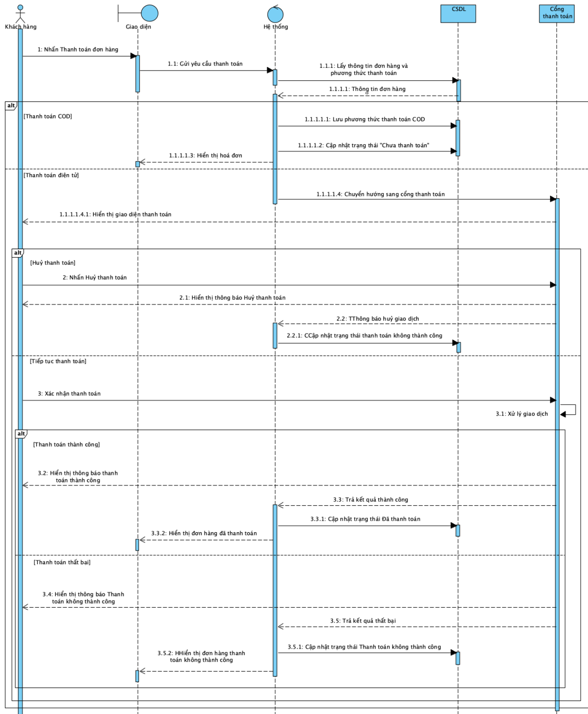
Hình 2.30: Biểu đồ tuần tự Thanh toán
