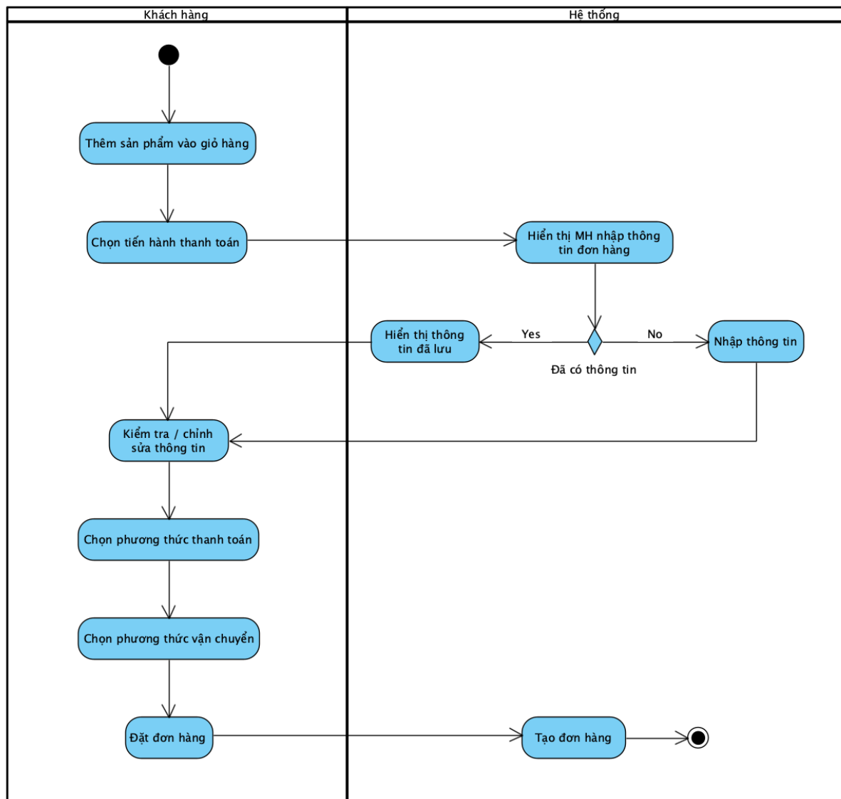
Hình 2.25: Biểu đồ hoạt động Đặt đơn hàng
