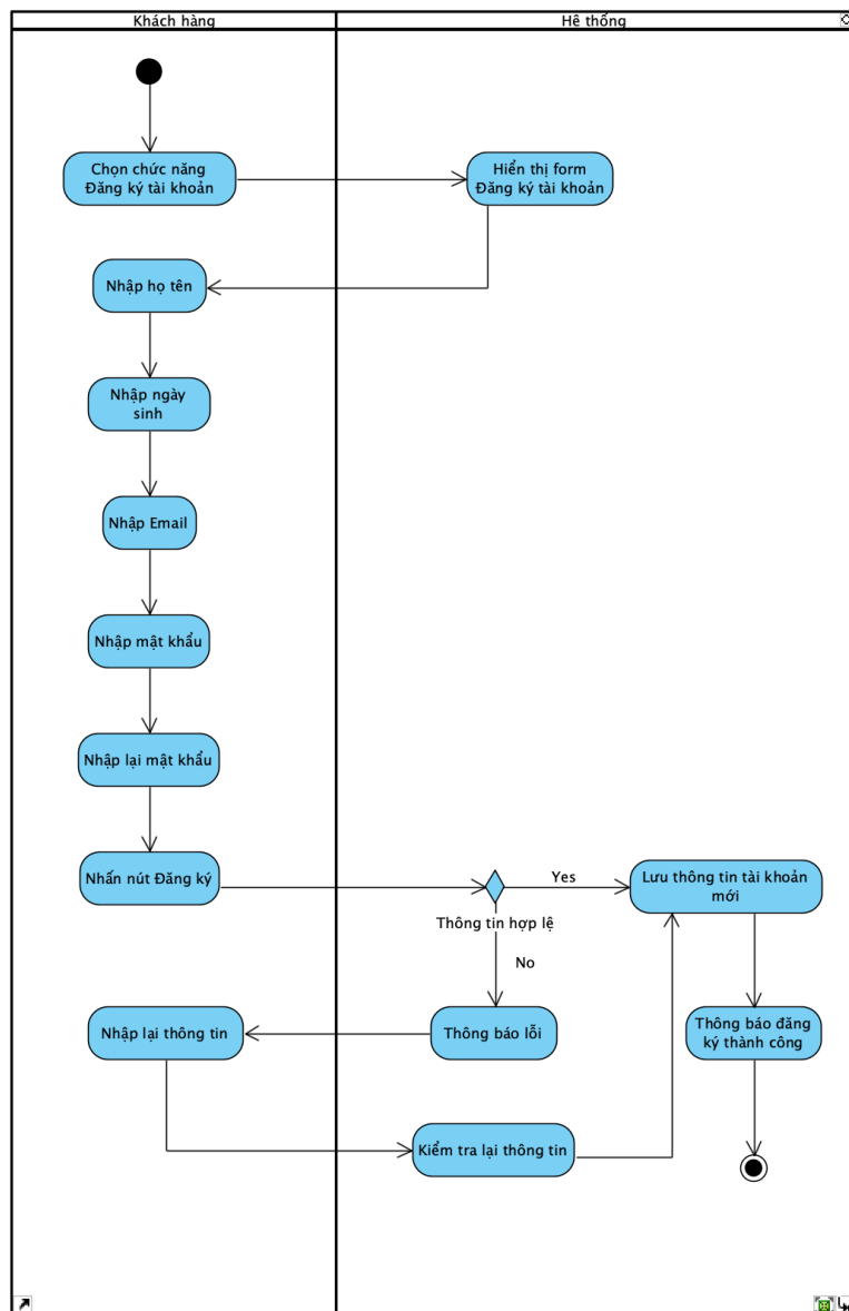
Hình 2.6: Biểu đồ hoạt động Đăng kí tài khoản
