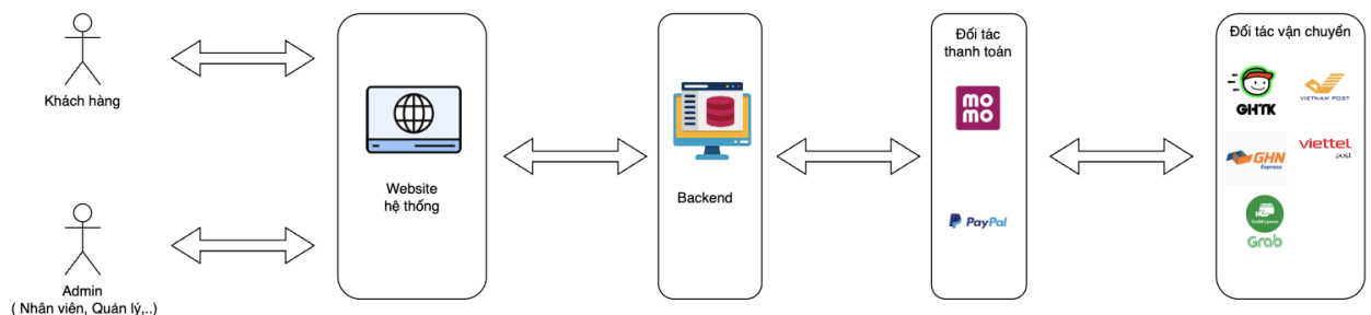
Hình 2.3: Sơ đồ tương tác giữa các thành phần trong hệ thống
