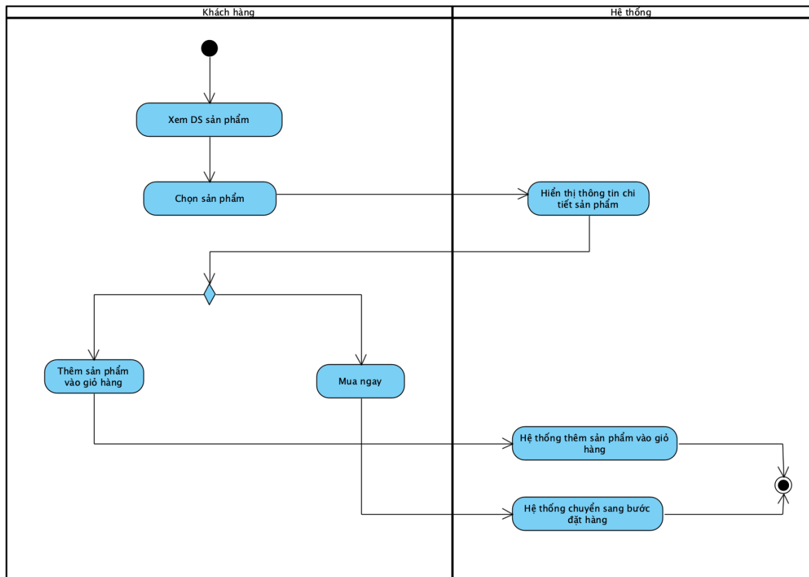
Hình 2.17: Biểu đồ hoạt động Xem chi tiết sản phẩm
