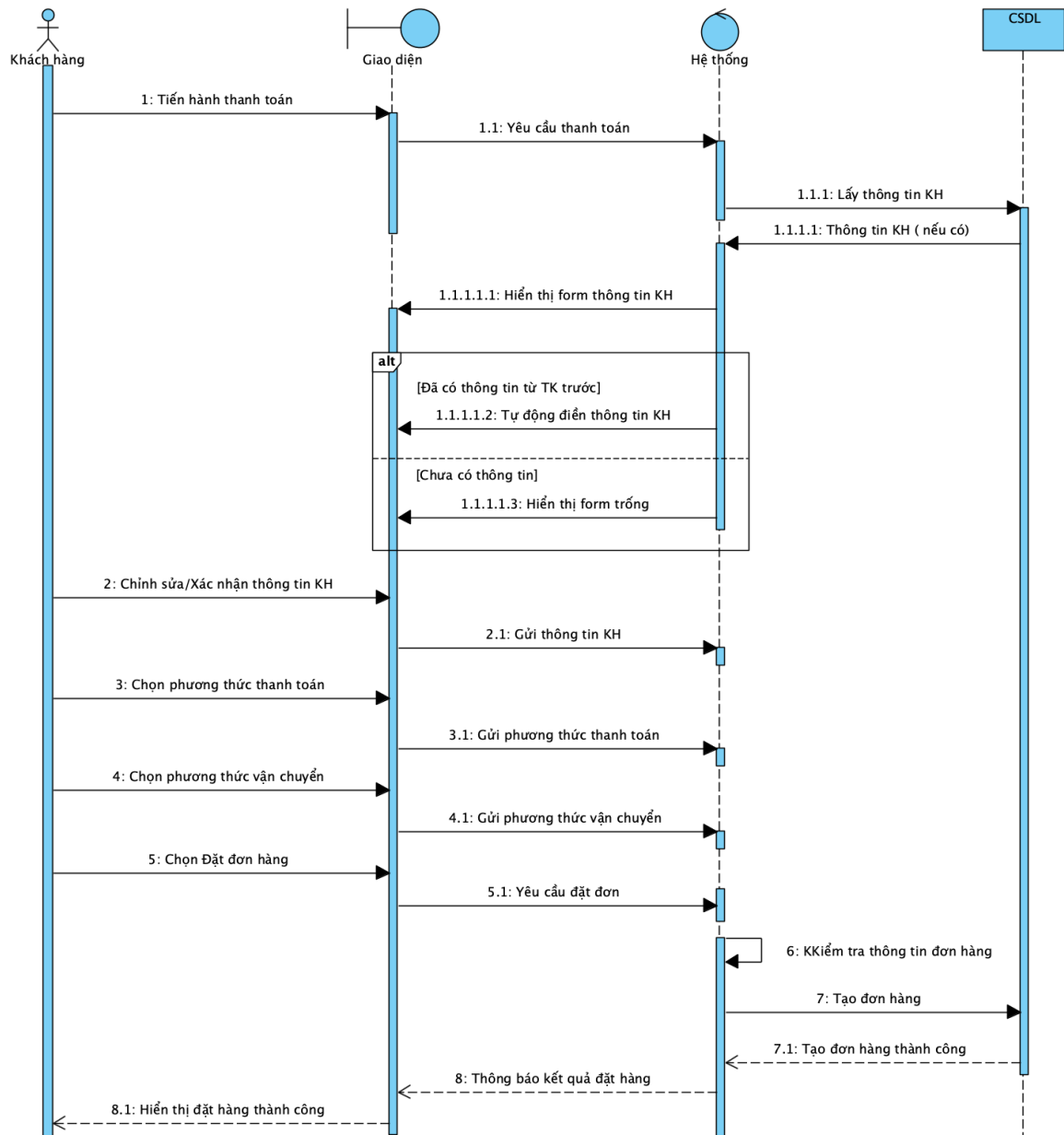
Hình 2.26: Biểu đồ tuần tự Đặt đơn hàng
