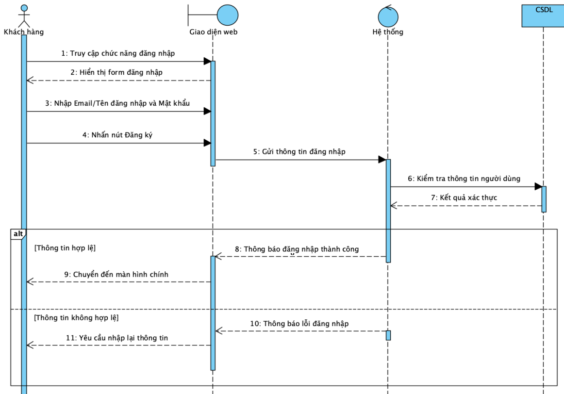
Hình 2.10: Biểu đồ tuần tự Đăng nhập tài khoản
