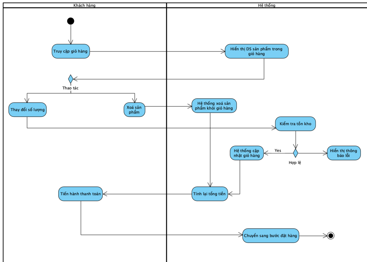
Hình 2.21: Biểu đồ hoạt động Quản lý giỏ hàng
