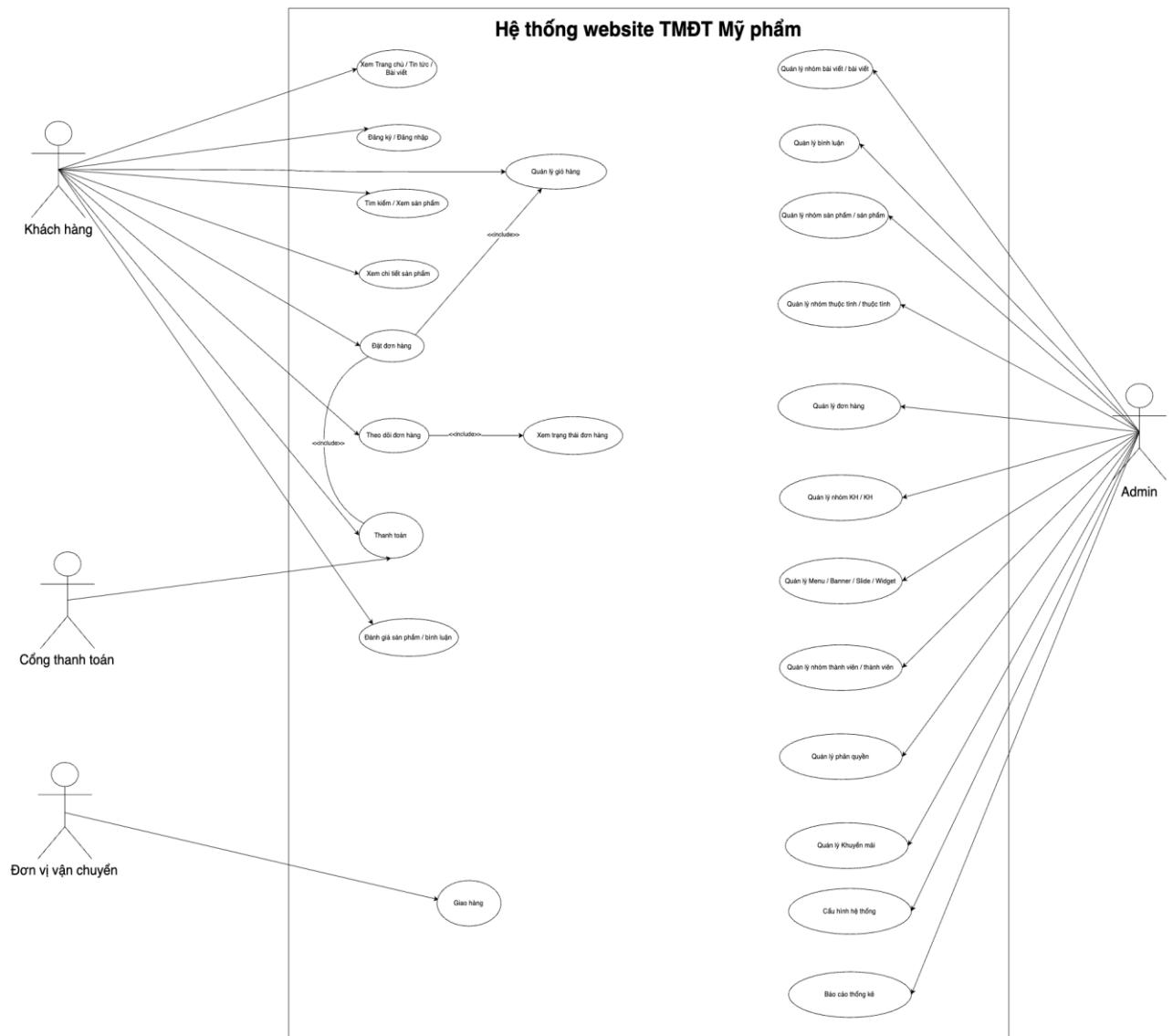
Hình 2.4: Biểu đồ Usecase tổng quát
