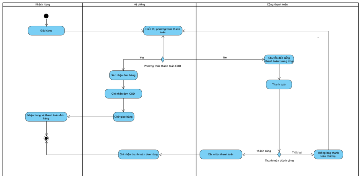
Hình 2.29: Biểu đồ hoạt động Thanh toán
