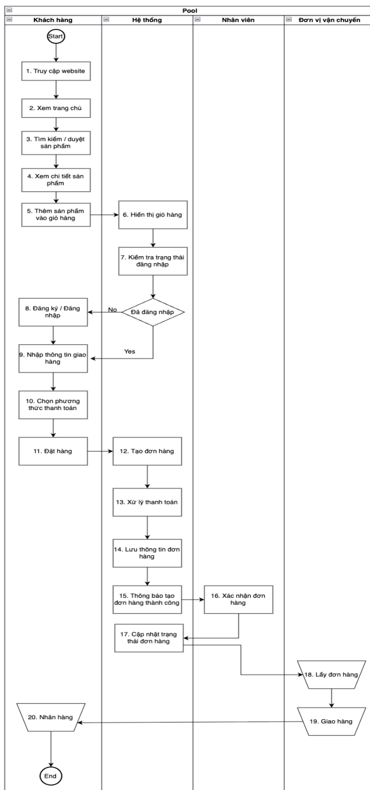
Hình 2.2: Quy trình nghiệp vụ mua hàng trên website
