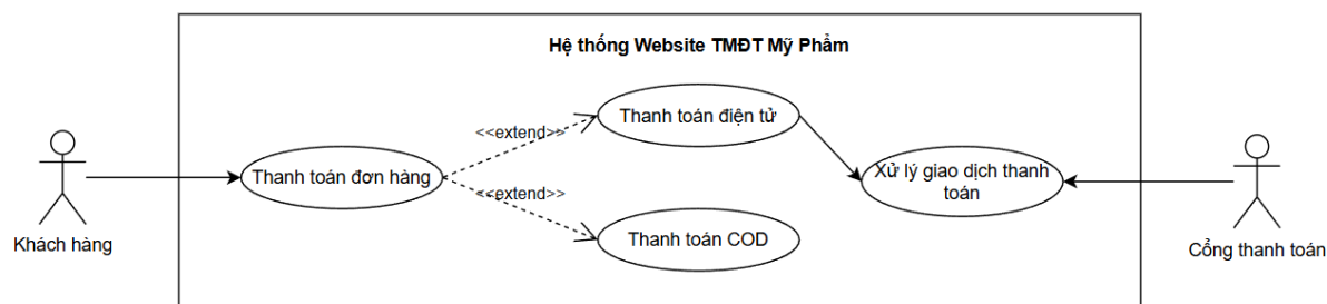
Hình 2.28: Biểu đồ Usecase Thanh toán
