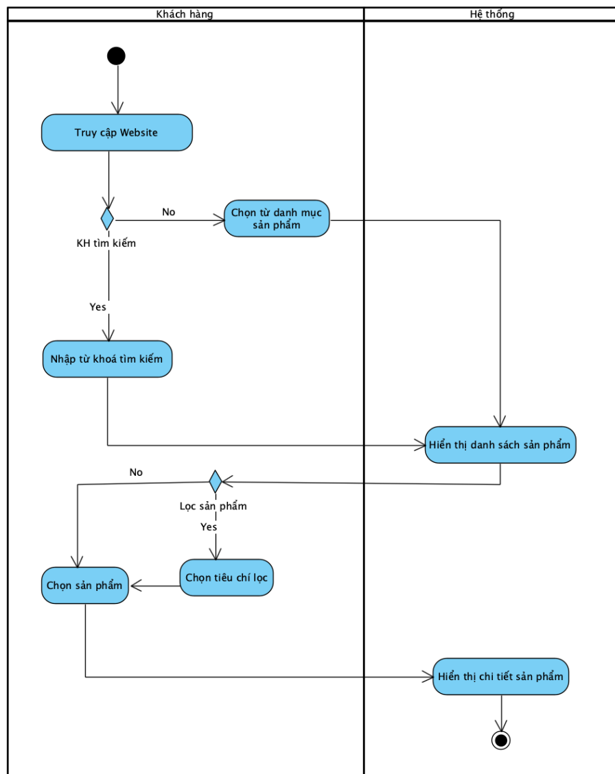
Hình 2.13: Biểu đồ hoạt động Tìm kiếm/ Xem danh sách sản phẩm
