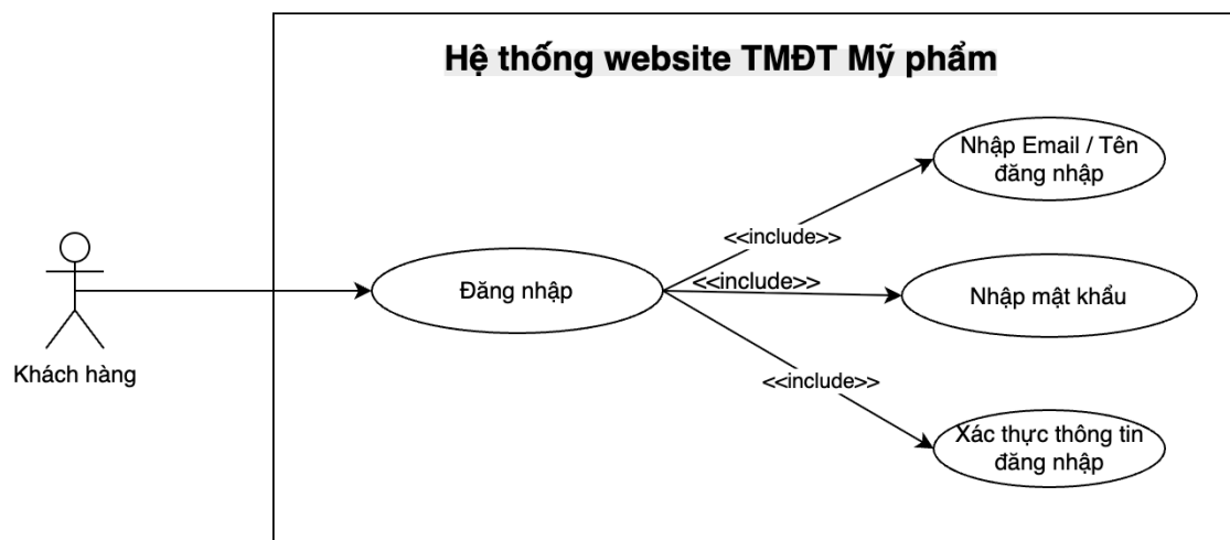
Hình 2.8: Biểu đồ Usecase Đăng nhập tài khoản
