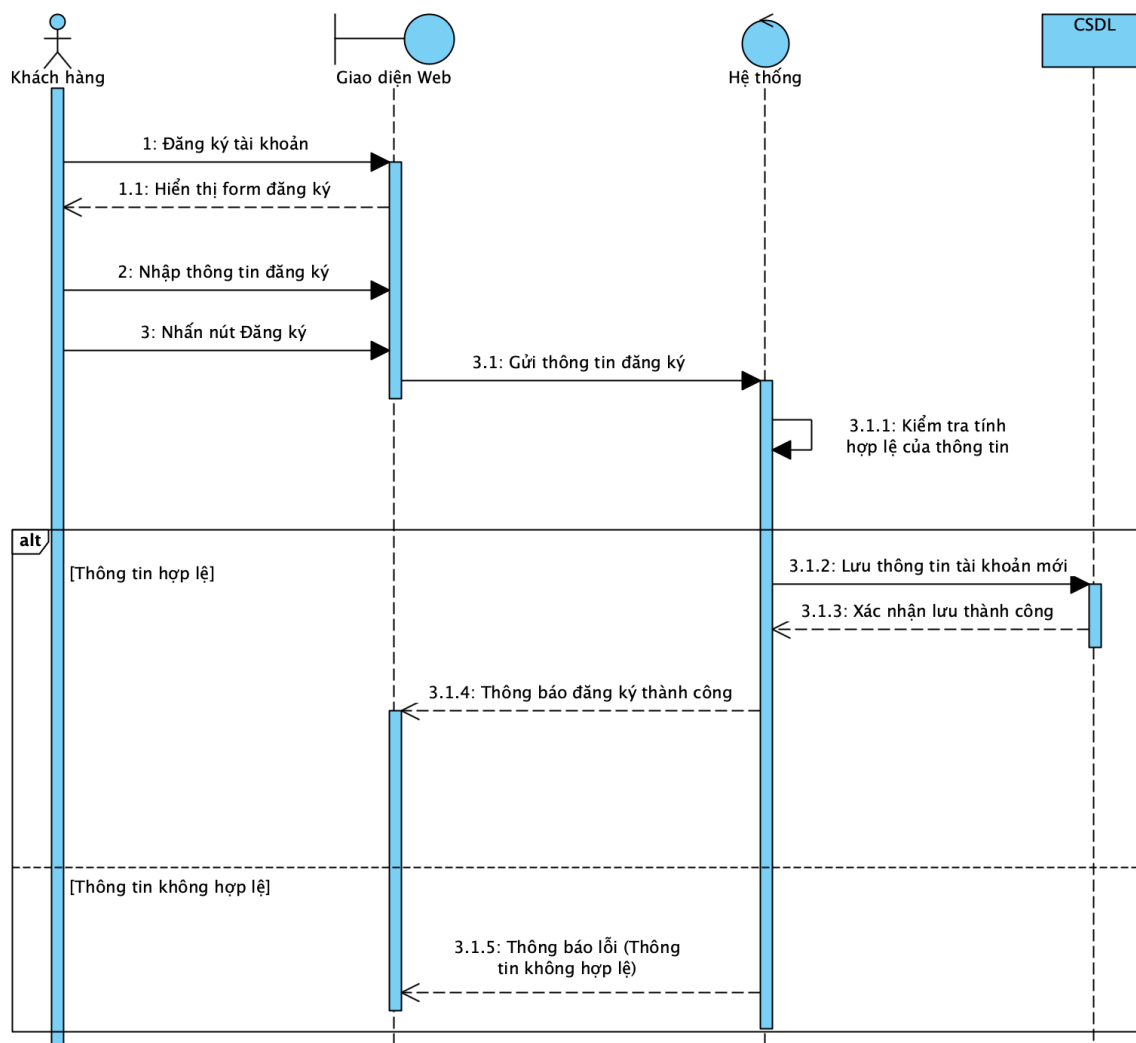
Bảng 2.7: Biểu đồ tuần tự Đăng kí tài khoản
