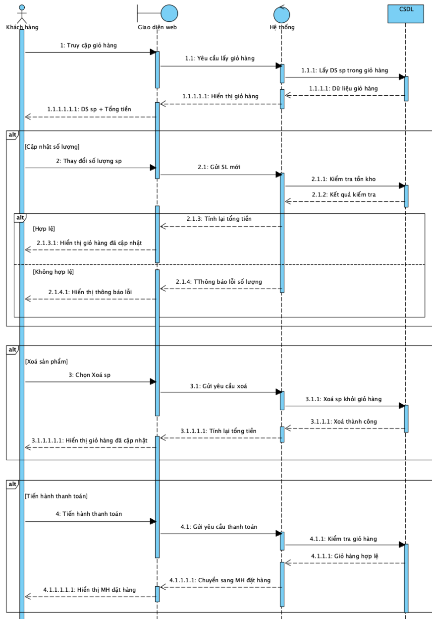
Hình 2.22: Biểu đồ tuần tự Quản lý giỏ hàng
