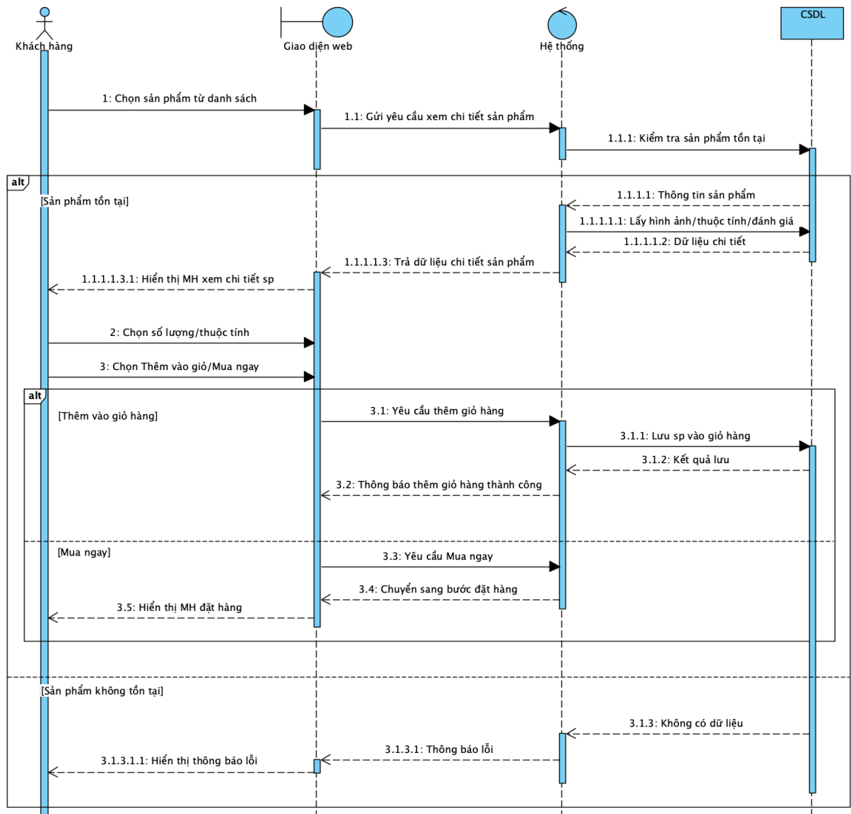
Hình 2.18: Biểu đồ tuần tự Xem chi tiết sản phẩm
