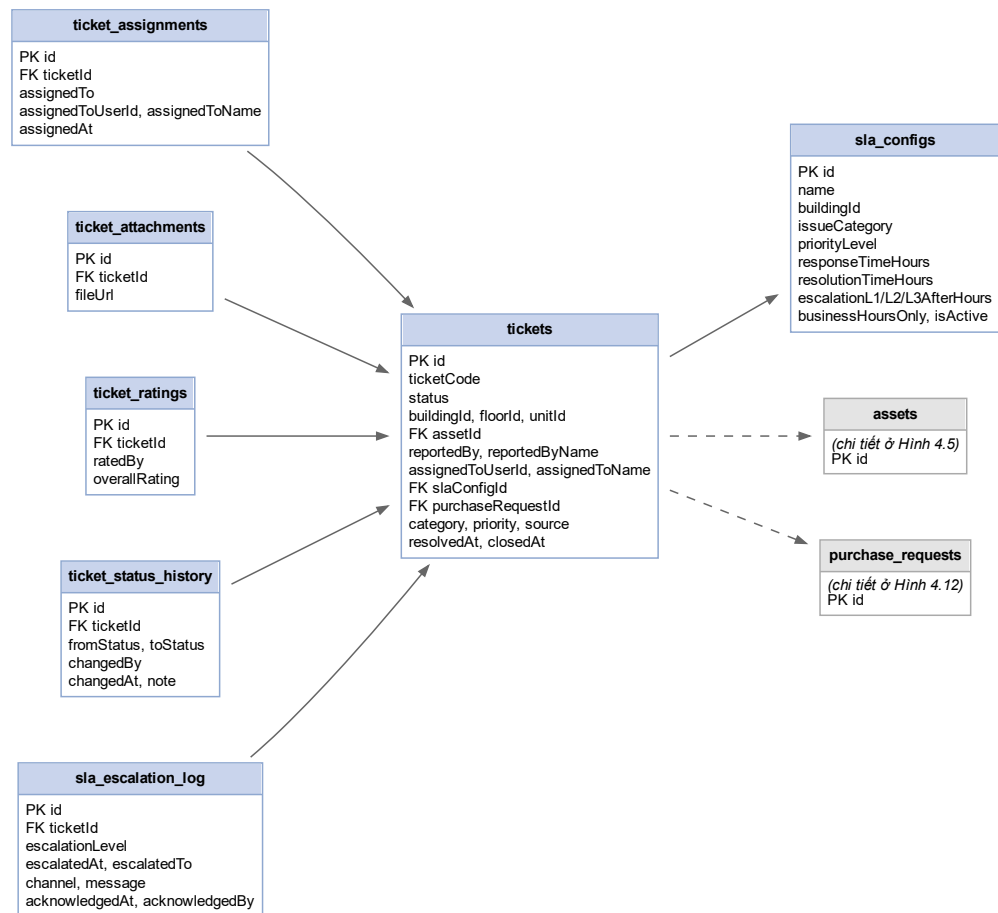
Hình 4.34. Sơ đồ thực thể – liên kết (ERD) phân hệ Quản lý sự cố & SLA
