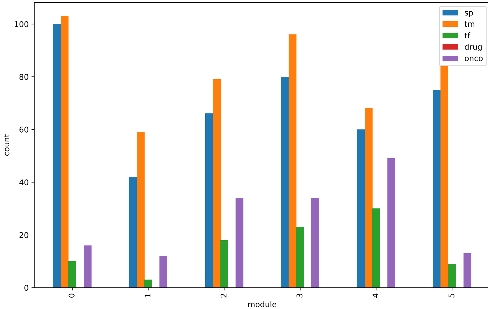
Annotation hits per module
