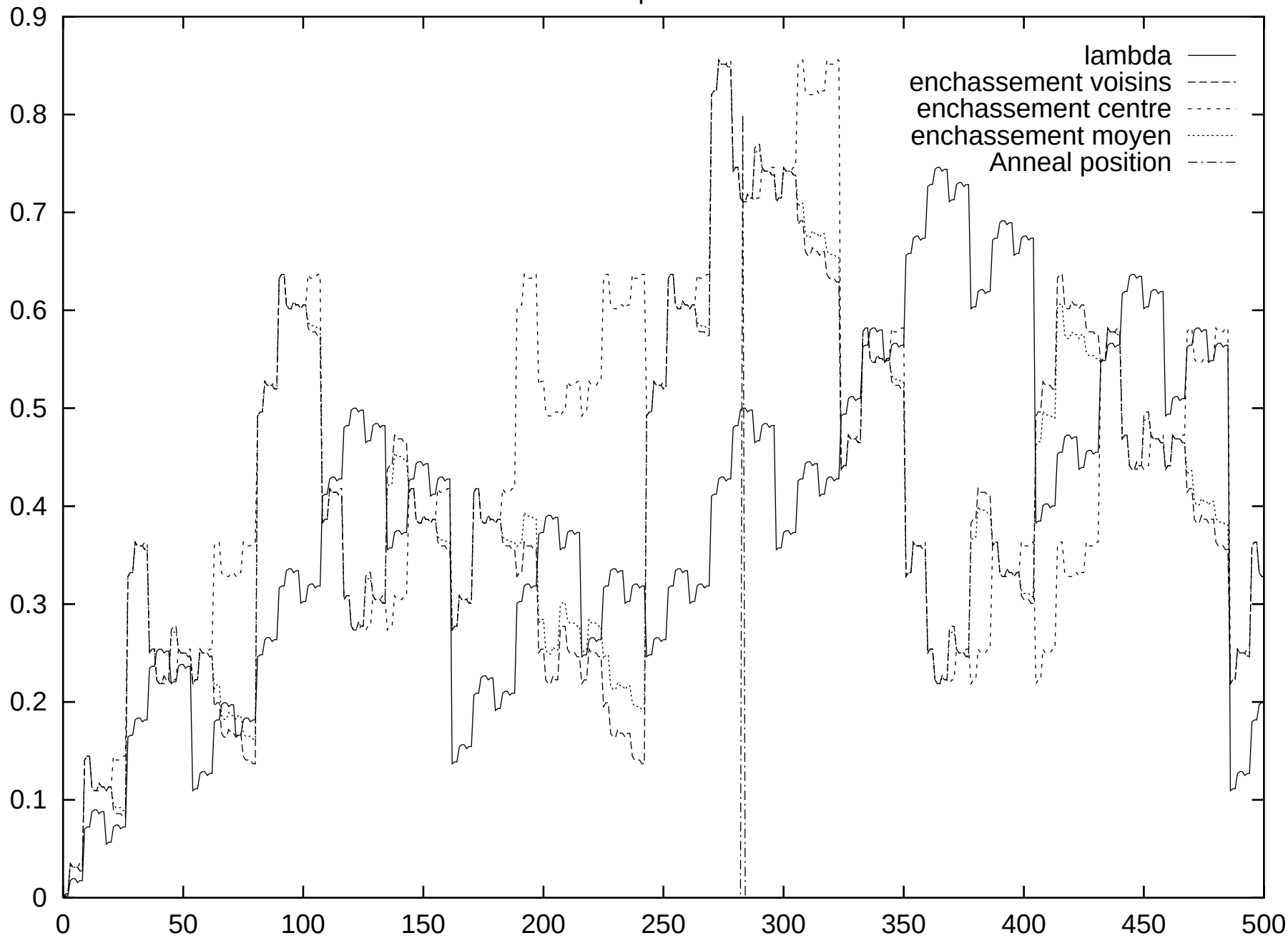
lambda et enchassement pour les 59049 CA additif 01U
