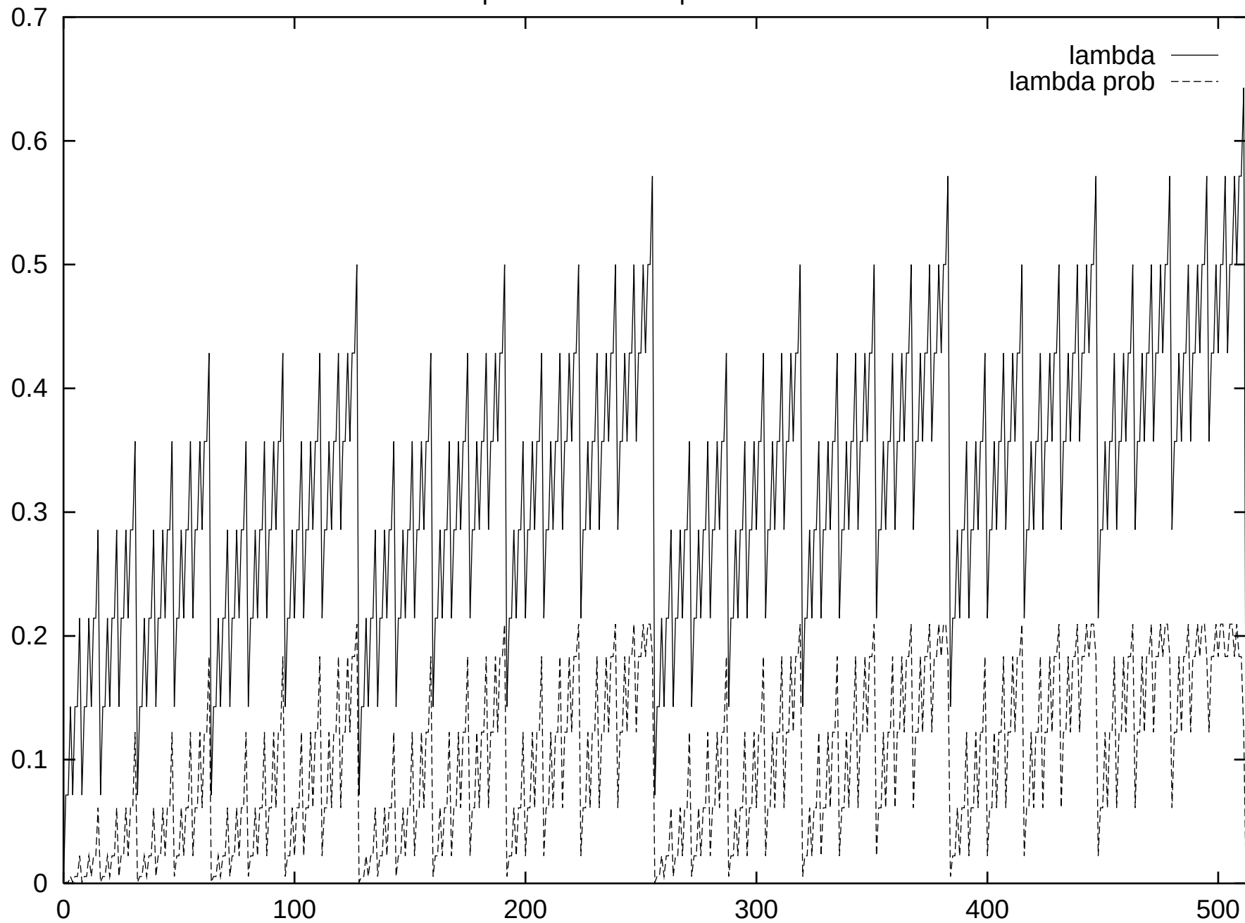
lambda et prob. de lambda pour 512/16384 entiers
