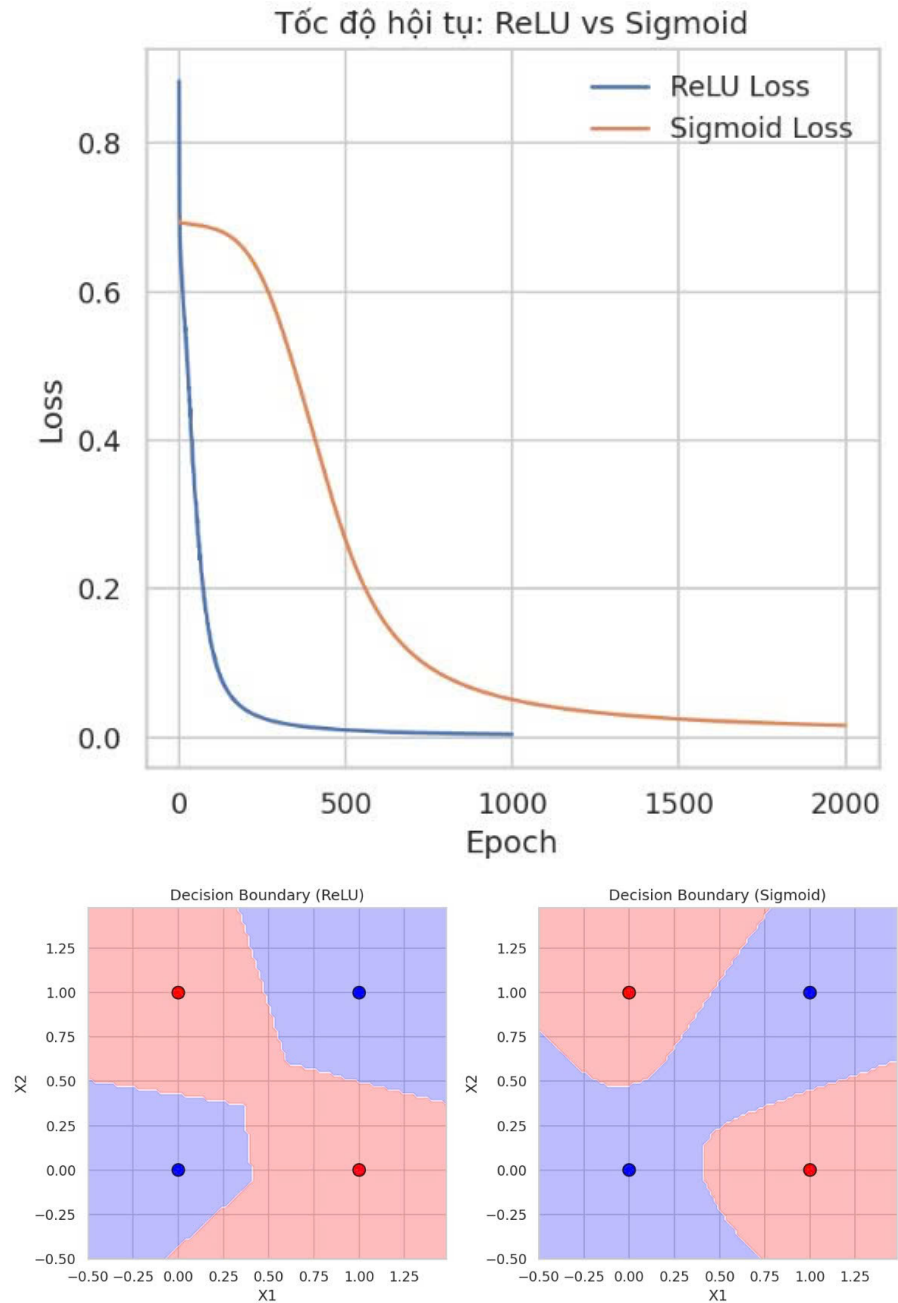
Hình 3.3: Tốc độ hội tụ và ranh giới quyết định của MLP trên bài toán XOR
