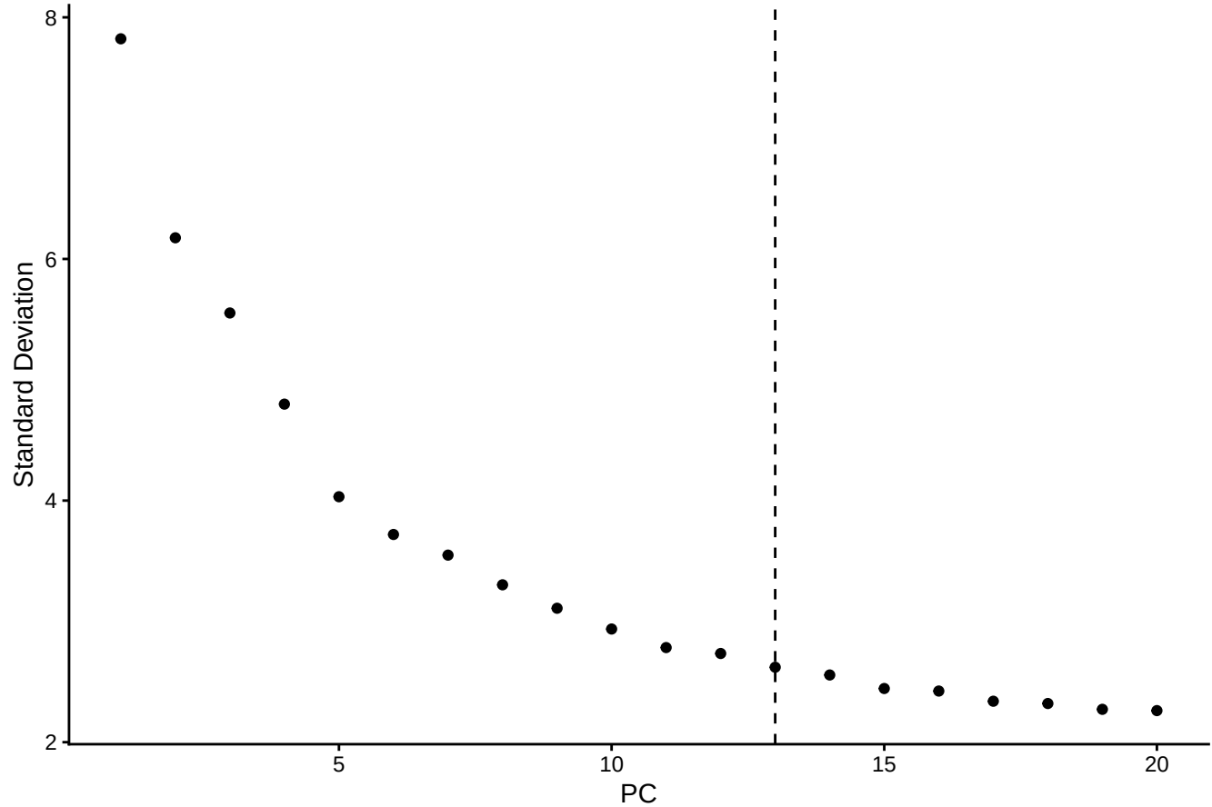
PCA elbow plot; PC 1:13 used downstream
