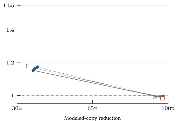
(b) LU
