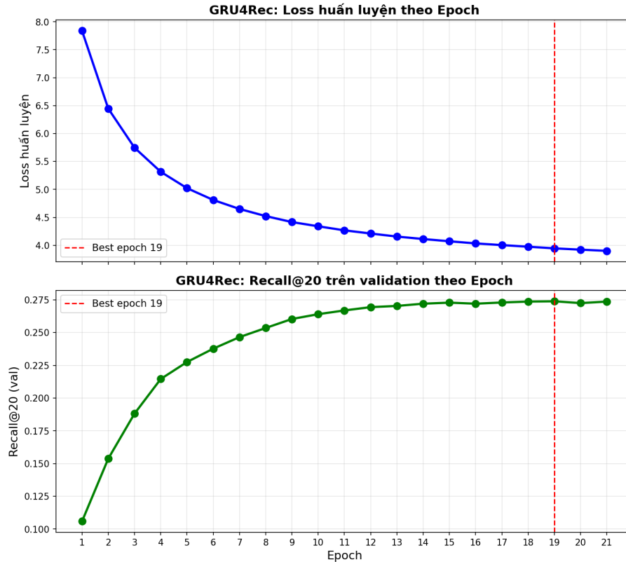
Hình 3.2: Loss huấn luyện và Recall@20 trên validation của GRU4Rec theo epoch; vạch đỏ là best epoch (19) do early stopping chọn. Nguồn: kết quả thực nghiệm của nhóm từ output/all_results.pkl , trực quan hóa bằng src/plots.py .
