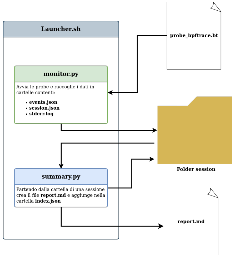
Figura 3.1: Architettura del sistema: flusso di dati tra probe bpfttrace, monitor.py, summary.py e launcher.sh.
