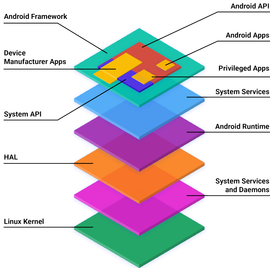
Figura 2.2: Architettura a livelli del sistema operativo Android.
