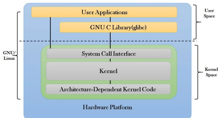
Figura 2.1: Architettura del sistema Linux: kernel space, user space e system call.
