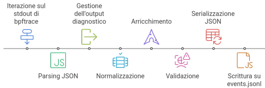
Figura 3.4: Pipeline di elaborazione degli eventi in monitor.py
