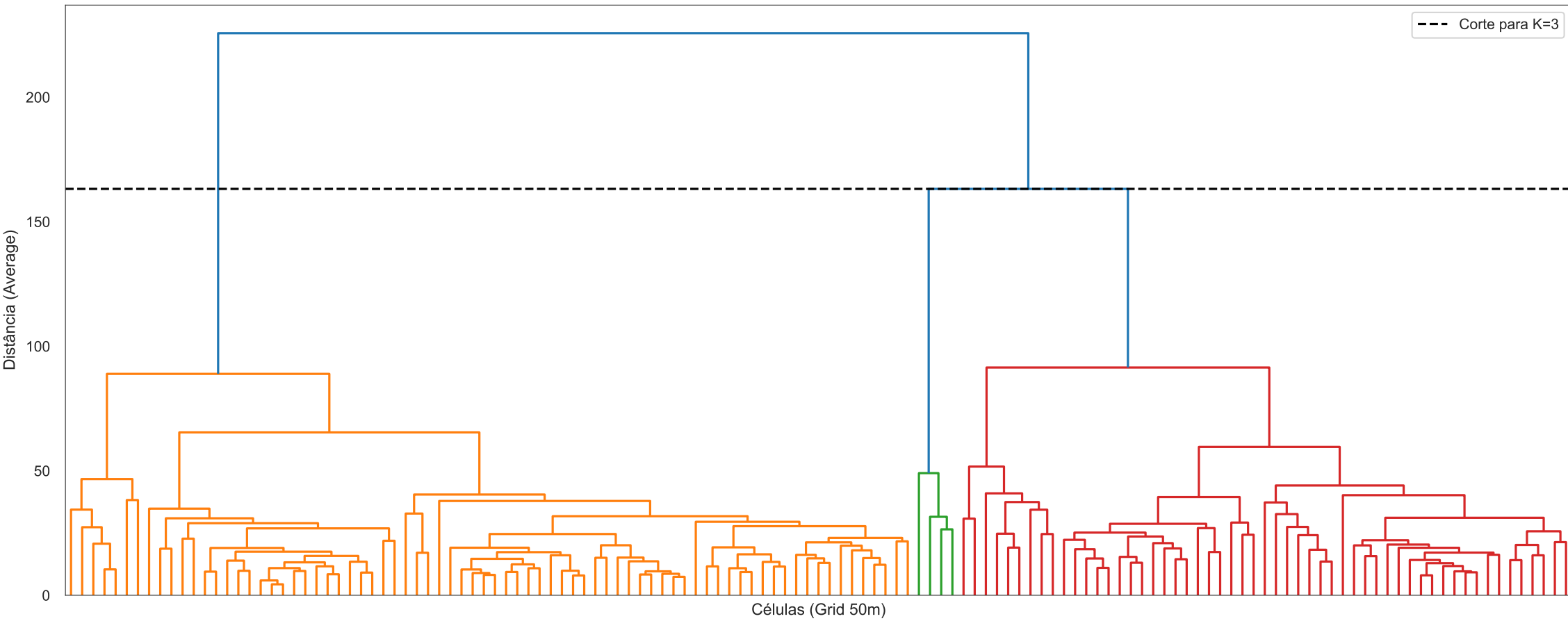
Dendrograma de Clustering Hierárquico (DTW) - K=3
