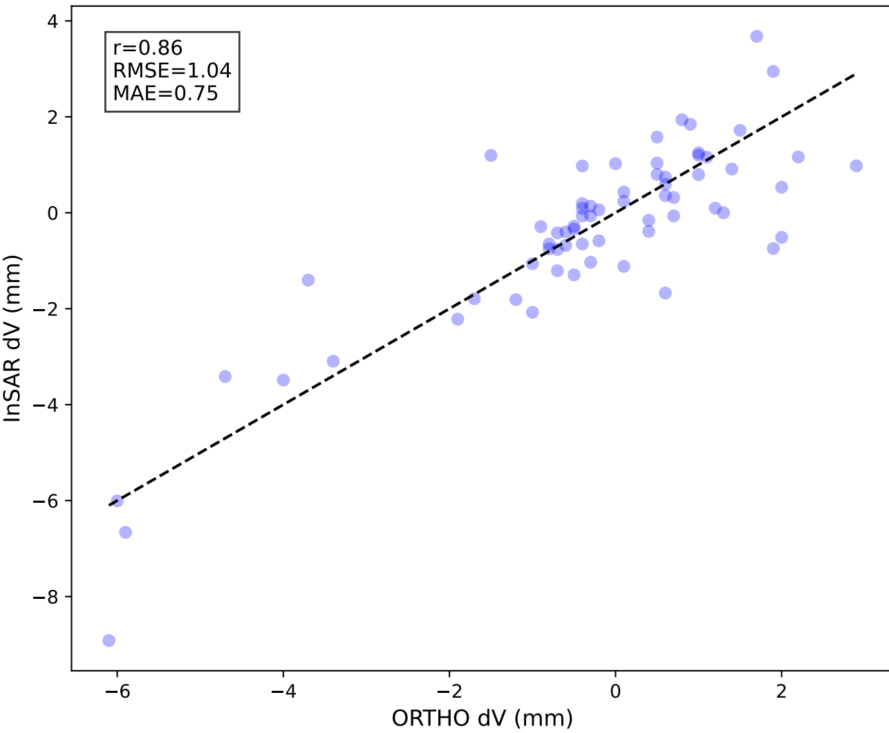
Comparação dV InSAR vs ORTHO
