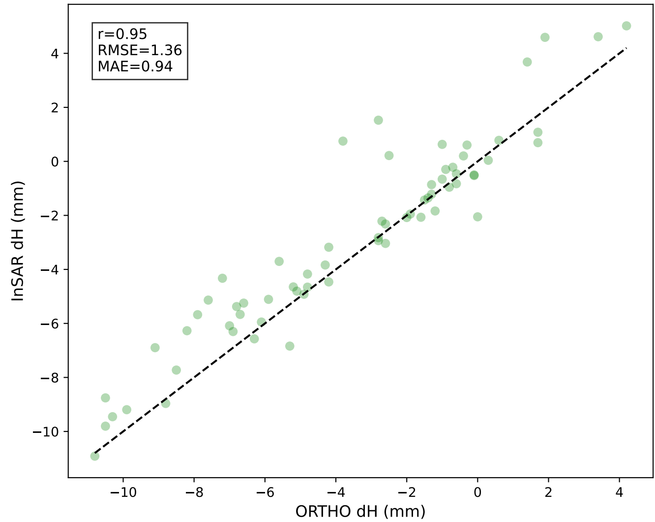
Comparação dH InSAR vs ORTHO
