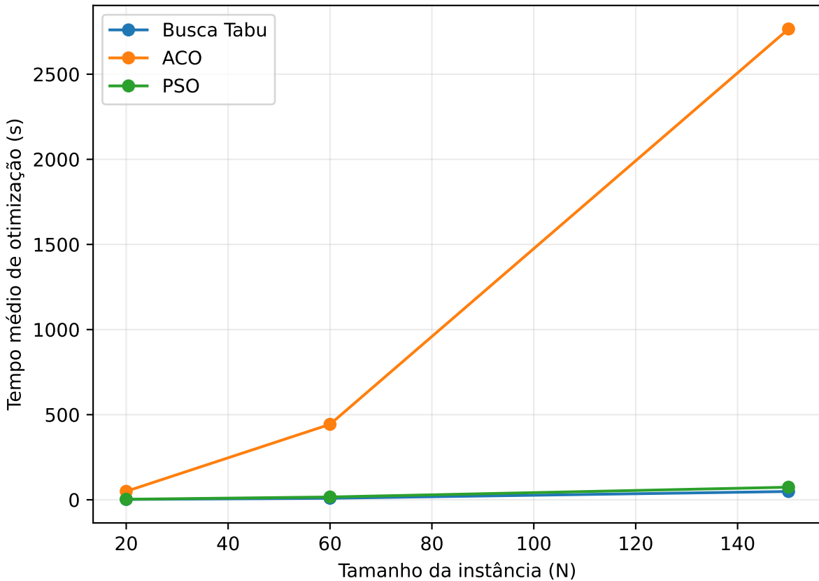
Escalabilidade — Tempo médio de otimização (s), K=5
