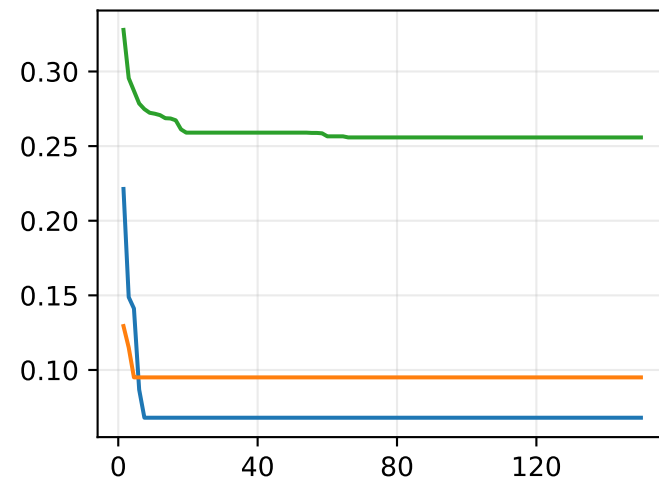
N=150, K=3
