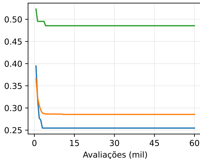
N=60, K=8
