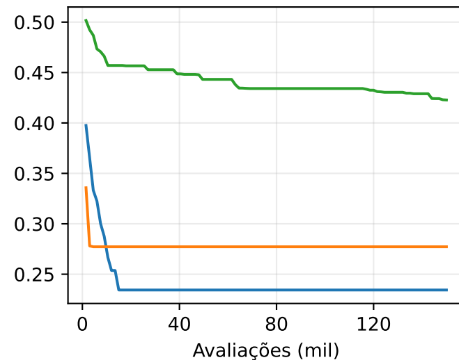
N=150, K=8
