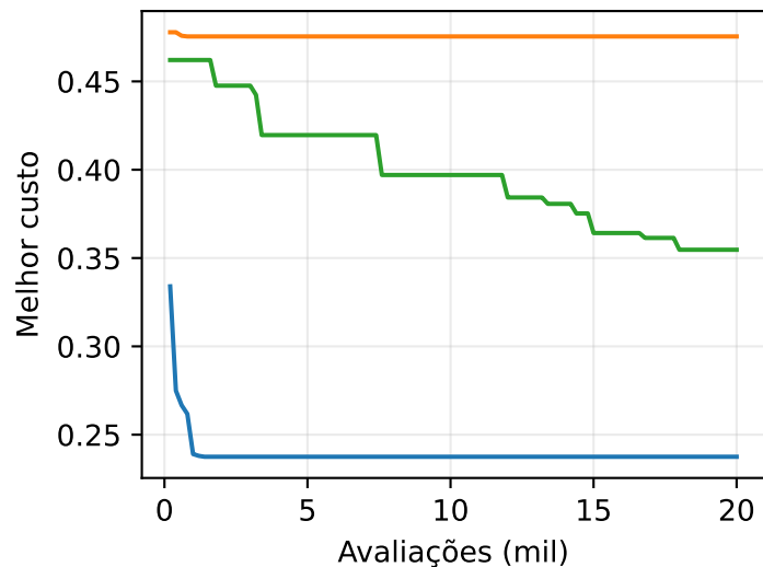
N=20, K=8
