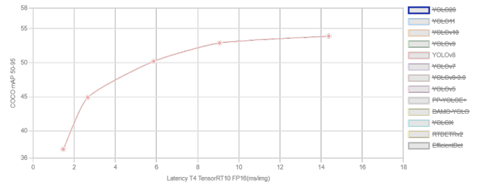
Fig. 2. Courbe de performance des différentes variantes du modèle YOLOv8. Source : Ultralytics ultralytics 'models
