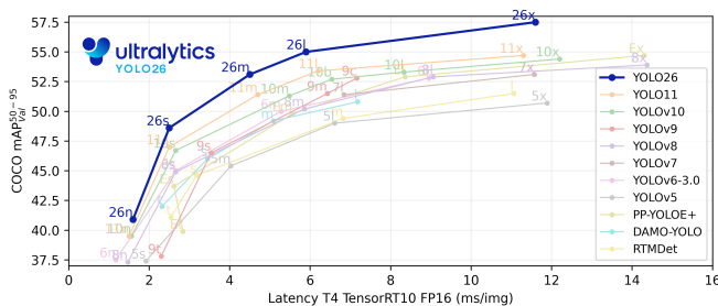
Fig. 1. Comparaison des modèles YOLO supportés par Ultralytics. Source : Ultralytics ultralytics.com/models
