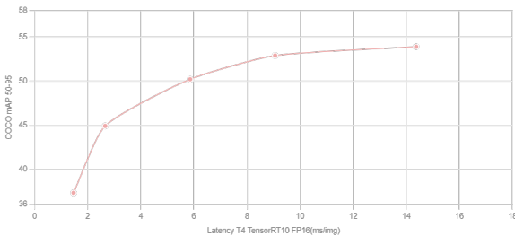
Fig. 6. Courbe de performance des différentes variantes du modèle YOLOv8. Source : Ultralytics ultralytics' models
