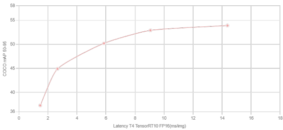
Fig. 6. Courbe de performance des différentes variantes du modèle YOLOv8. Source : Ultralytics[19]
