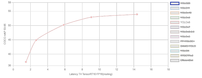
Fig. 2. Courbe de performance des différentes variantes du modèle YOLOv8. Source : Ultralytics[18]
