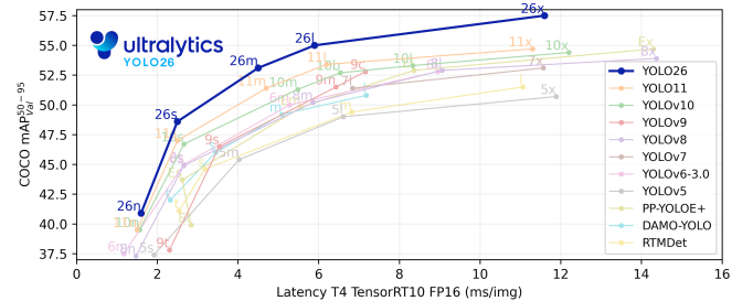
Fig. 2. Comparaison des modèles YOLO supportés par Ultralytics. Source : Ultralytics[18]
