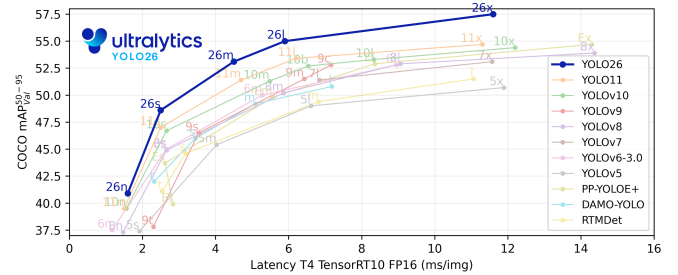
Fig. 1. Comparaison des modèles YOLO supportés par Ultralytics. Source : Ultralytics [10]
