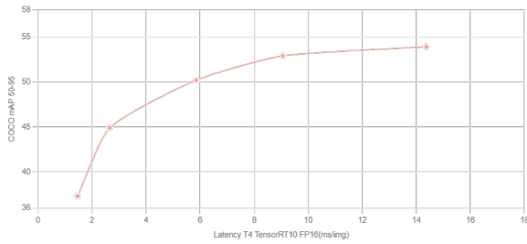
Fig. 2. Courbe de performance des différentes variantes du modèle YOLOv8. Source : Ultralytics [10]
