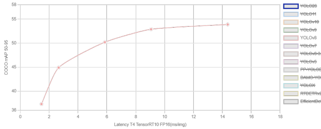
Fig. 6. Courbe de performance des différentes variantes du modèle YOLOv8. Source : Ultralytics[18]
