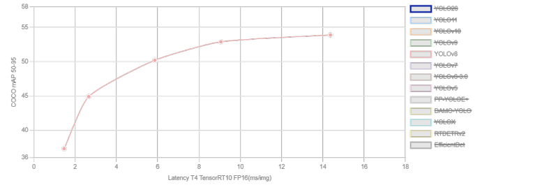
Fig. 6. Courbe de performance des différentes variantes du modèle YOLOv8. Source : Ultralytics[18]
