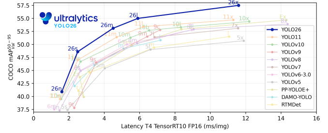
Fig. 5. Comparaison des modèles YOLO supportés par Ultralytics. Source : Ultralytics[18]
