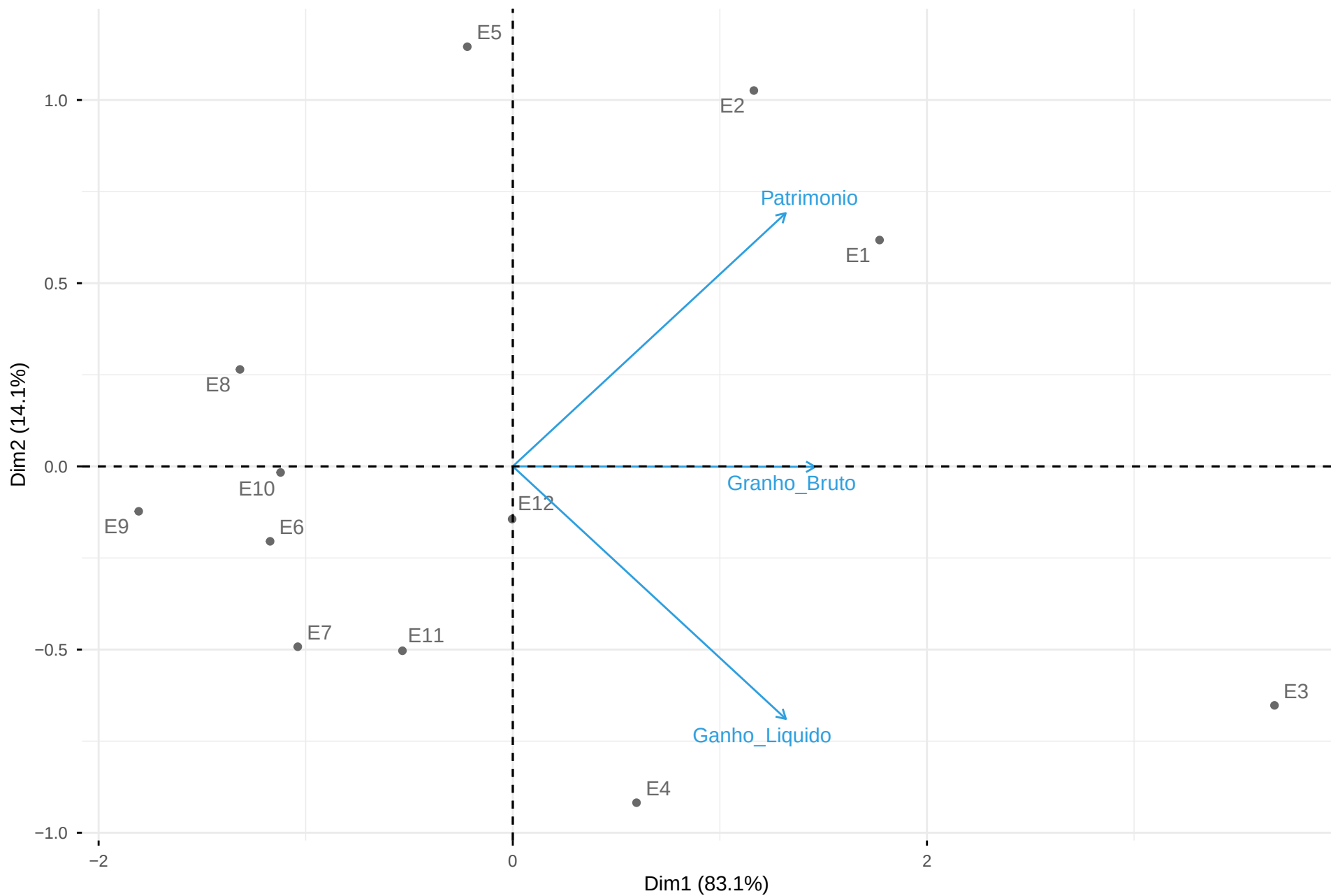
PCA – Biplot
